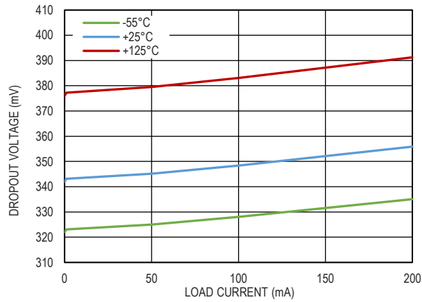
图 12. 压差电压和负载电流的关系, V OUT =3.0V
