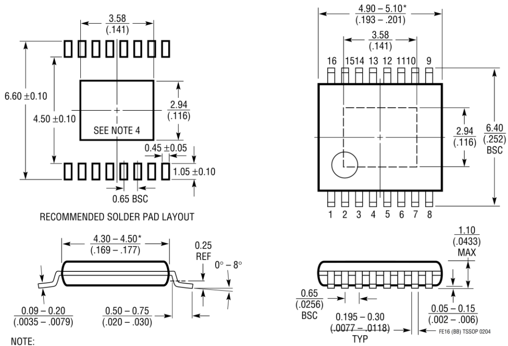
图 24. 16 引脚 TSSOP
