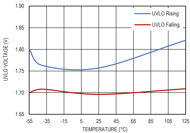
图 15. UVLO 阈值
