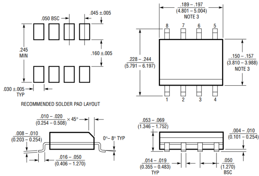
图 23. 8 引脚 SOIC-8
