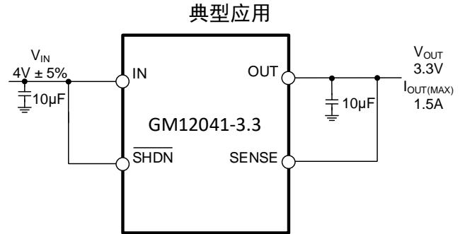
图 1 典型应用
