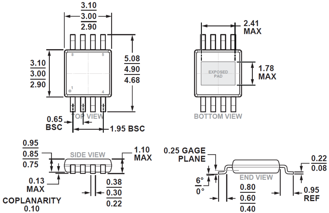
图 35.8 引脚 MSOP
