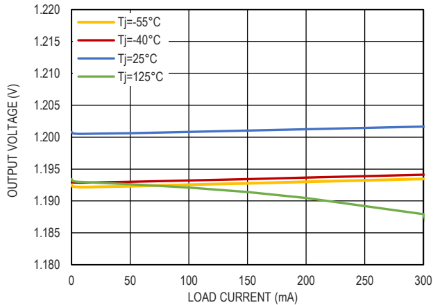
图 12. 1.2V 输出电压和负载电流的关系
