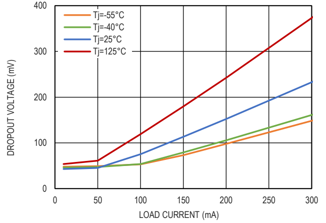
图 9. 5.0V 压差电压和负载电流的关系
