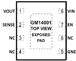
图 3.8 引脚 DFN 的引脚配置
