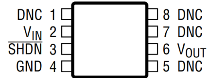
图 1. 8 引脚 MSOP
