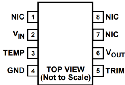
图 4. SO-8 引脚配置(顶视图)
