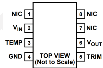
图 2. 8 引脚 SOIC
