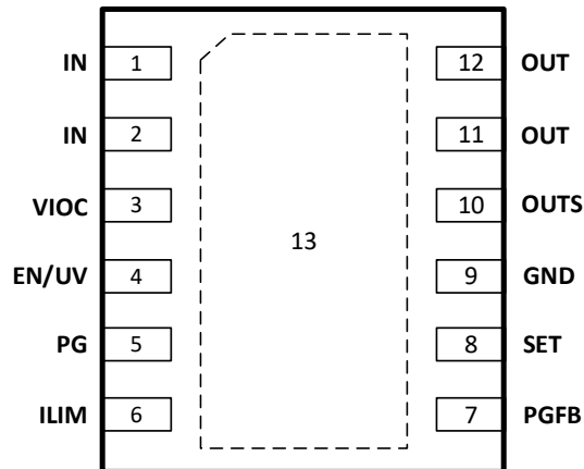
图 6. GM1205ACPZ-1 引脚配置(顶视图)
