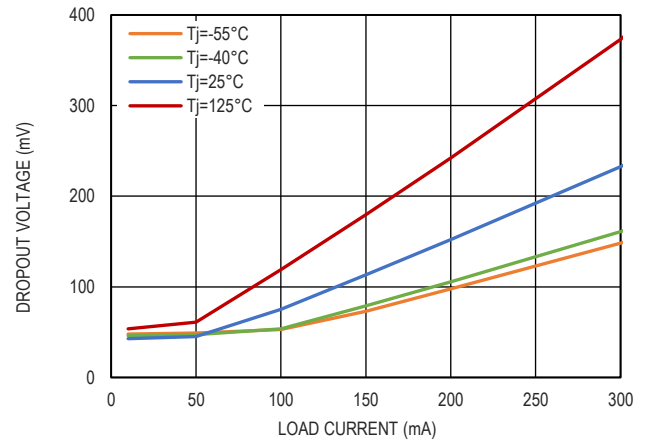
图 8. 5.0V 压差电压和负载电流的关系
