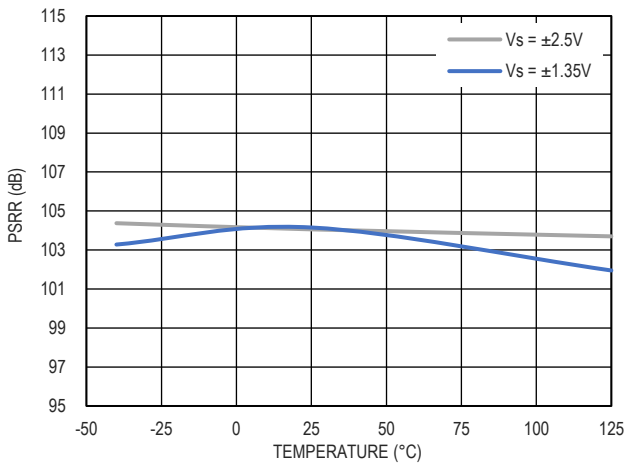
图 13. 大信号 PSRR vs. Temperature
