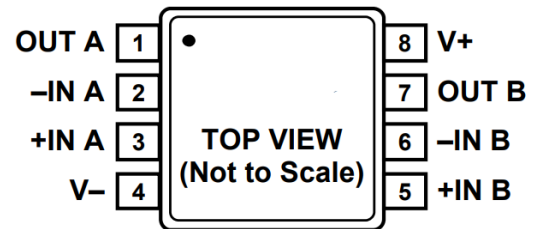
图 1. 8 引脚 MSOP 和 SOP
