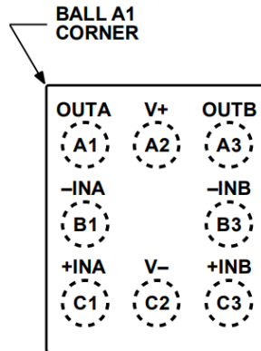
图 4. 8 引脚 WLCSP (顶视图)
