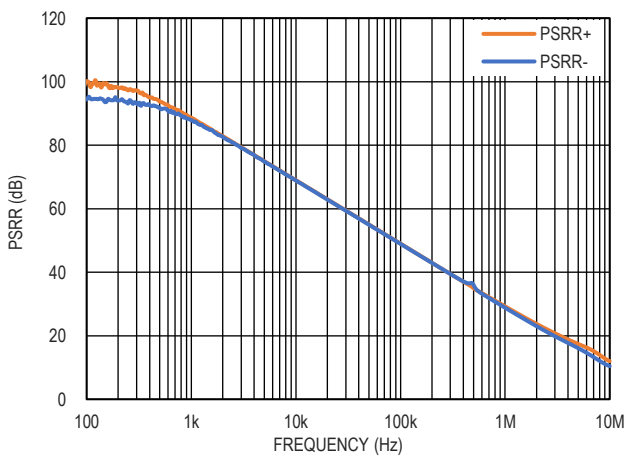
图 16. PSRR vs. Frequency, V_S=\pm 2.5V , V_{IN}=50mV , R_L=1M\Omega , C_L=47pF
