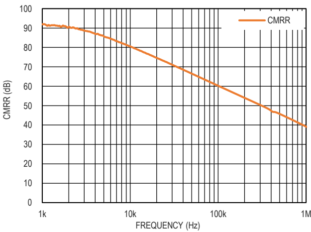
图 15. CMRR vs. Frequency, V_{IN}=28mV , R_L=1M\Omega , C_L=47pF
