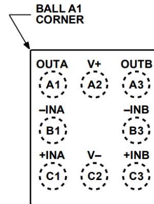
图 2. 8-Ball WLCSP
