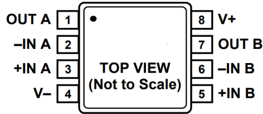
图 3. MSOP-8 和 SOP-8 引脚配置(顶视图)
