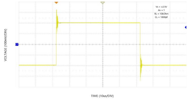
图 29. 驱动电容性负载
