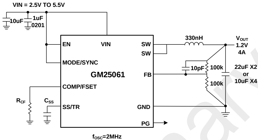
图 27. 2MHz, V_{IN}=3.3\text{V} , V_{OUT}=1.2\text{V} , I_{LOAD}=4\text{A}
