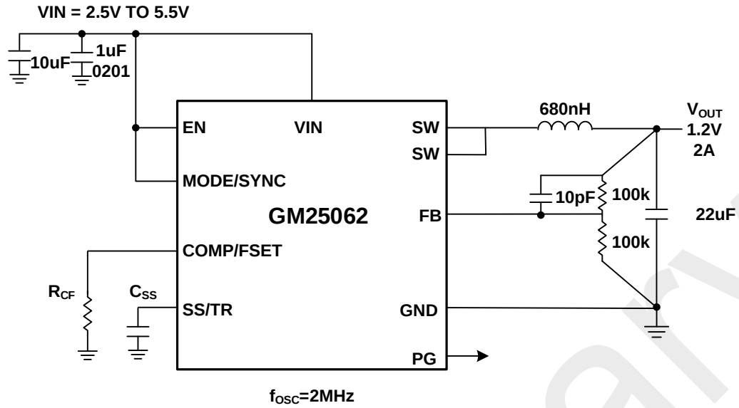
图 29. 2MHz, V_{IN}=3.3\text{V} , V_{OUT}=1.2\text{V} , I_{LOAD}=2\text{A}
