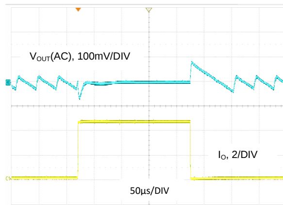
图 24. V_{OUT} = 1.2V , I_O = 0.1A 至 4.5A , 低功耗模式
