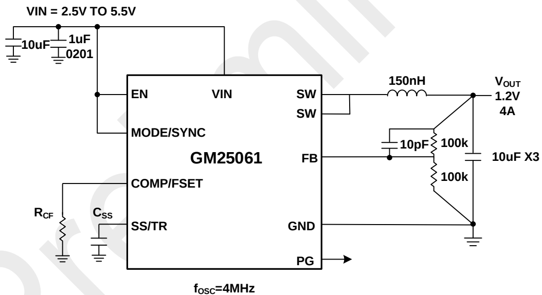
图 28. 4MHz, V_{IN}=3.3\text{V} , V_{OUT}=1.2\text{V} , I_{LOAD}=4\text{A}
