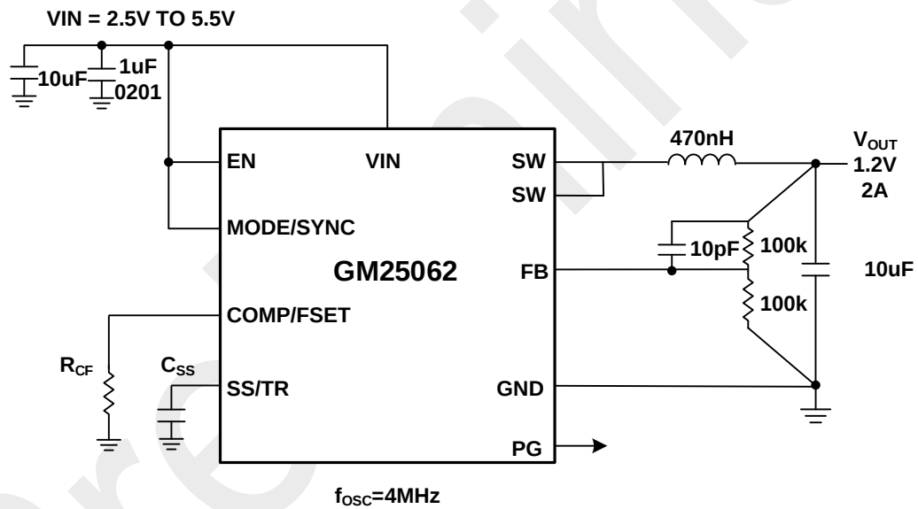
图 30. 4MHz, V_{IN}=3.3\text{V} , V_{OUT}=1.2\text{V} , I_{LOAD}=2\text{A}
