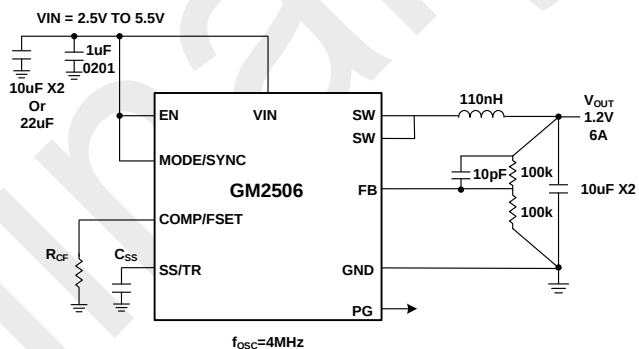
图 2. 4MHz 典型应用
