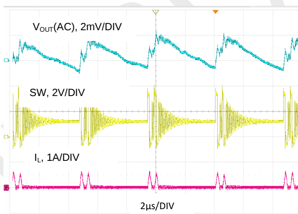
图 20. V_{OUT} = 1.2V , I_O = 100mA , PSM 模式
