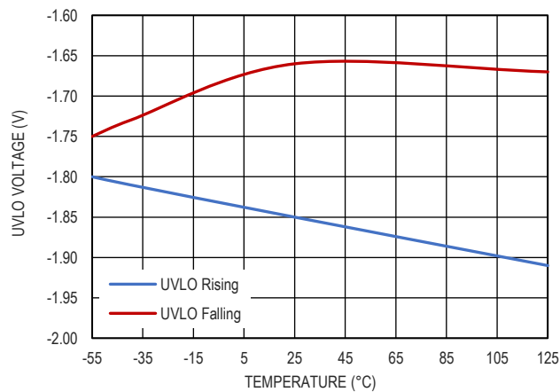
图 13. UVLO 阈值和结温的关系
