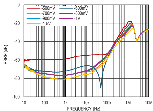
图 11. PSRR 和压差的关系, I_o = 200\text{mA}
