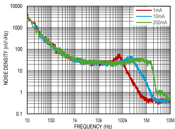
图 10. 噪声谱密度
