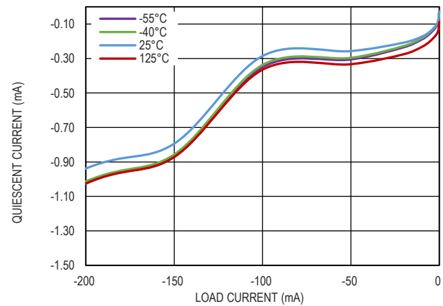
图 7. 静态电流与负载电流的关系
