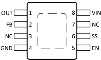
图 6. MSOP 引脚配置(顶视图)
