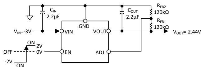
图 23. 设置可调输出电压
