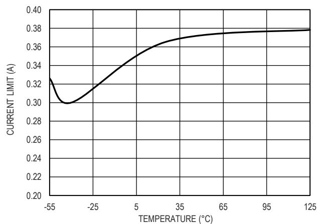
图 18. 限流值和结温的关系
