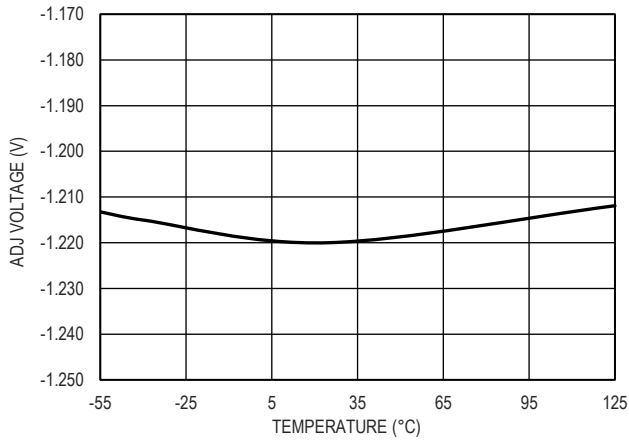
图 7. ADJ 引脚电压与结温 ( T_J ) 的关系
