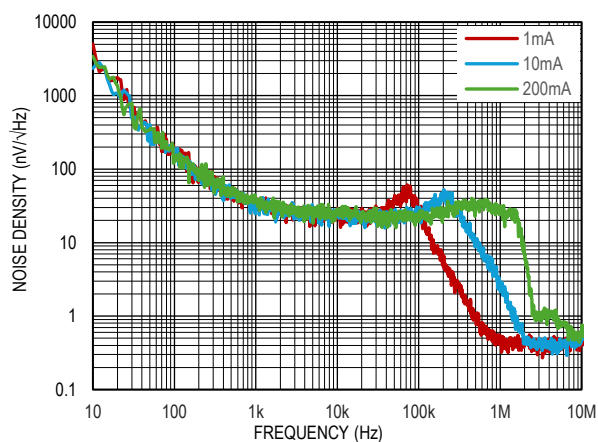
图 13. 噪声谱密度
