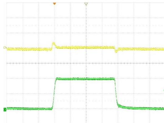
图 20. 负载瞬态响应, V_{IN} = -6V , V_{OUT} = -5V , I_O = -10 至 -200mA
