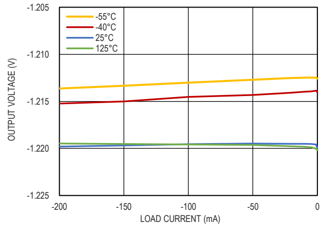
图 8. ADJ 引脚电压与 vs. 负载电流的关系
