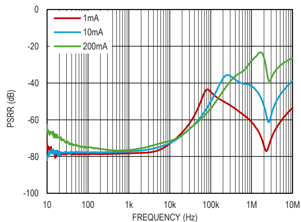
图 15. PSRR 和负载电流的关系
