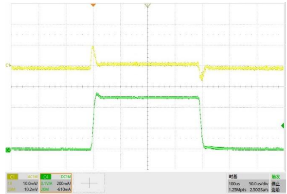
图 19. 负载瞬态响应, V_{OUT} = -5V , I_O = -10mA 至 -500mA
