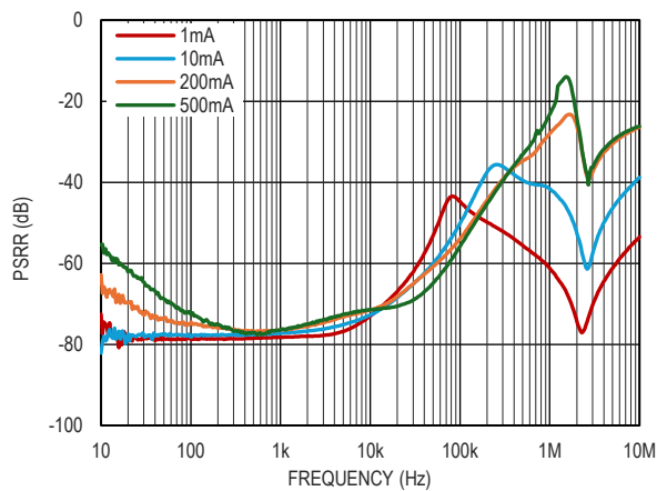
图 14. PSRR 和负载电流的关系
