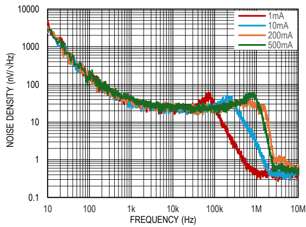
图 12. 噪声谱密度
