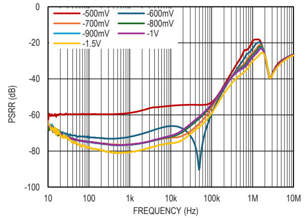
图 13. PSRR 和压差的关系, I_O = 200\text{mA}
