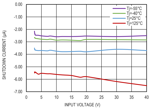
图 10. 静态电流与输入电压的关系
