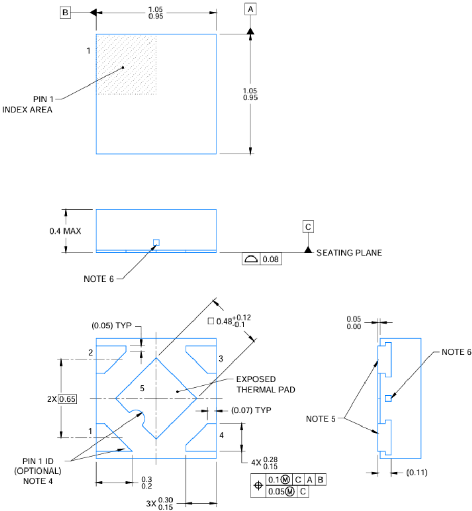
图 26.4 脚 DFN-4
