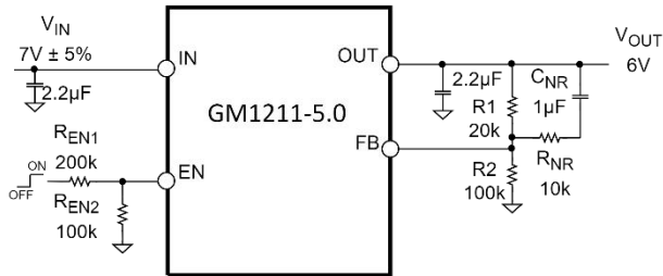
图 26. 噪声优化
