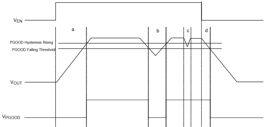
图 32 .PG 触发场景具有不同的运行状态
