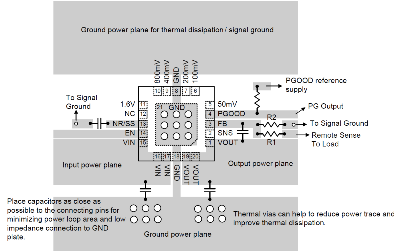
图 34. GM1203-1 布局示例
