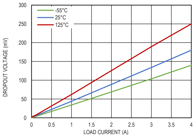
图 12. 压差电压和负载的关系, V_{OUT} = 5.0V , BIAS 浮空
