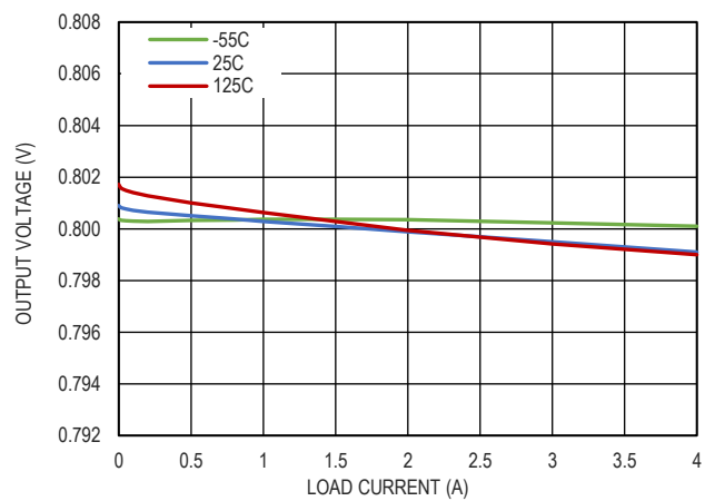
图 27. 负载调整率, BIAS 浮空
