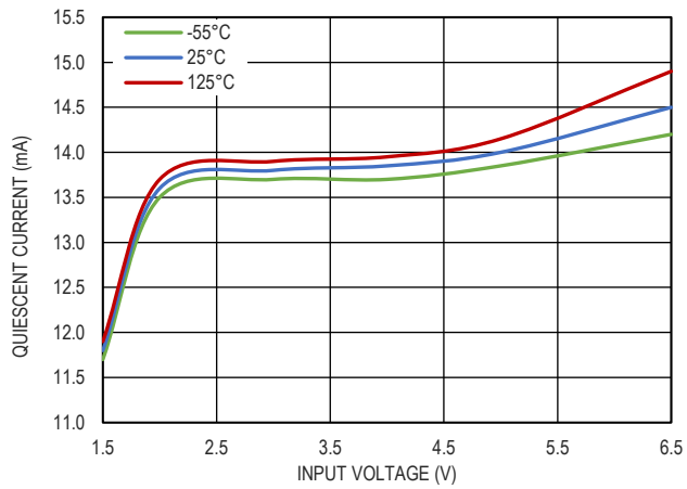
图 14. 静态电流和输入电压的关系, I_{OUT}=1mA
