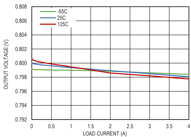
图 28. 负载调整率, V_{BIAS} = 5V
