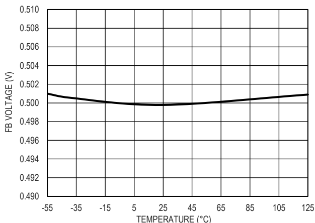
图 8. FB 引脚电压和温度的关系
