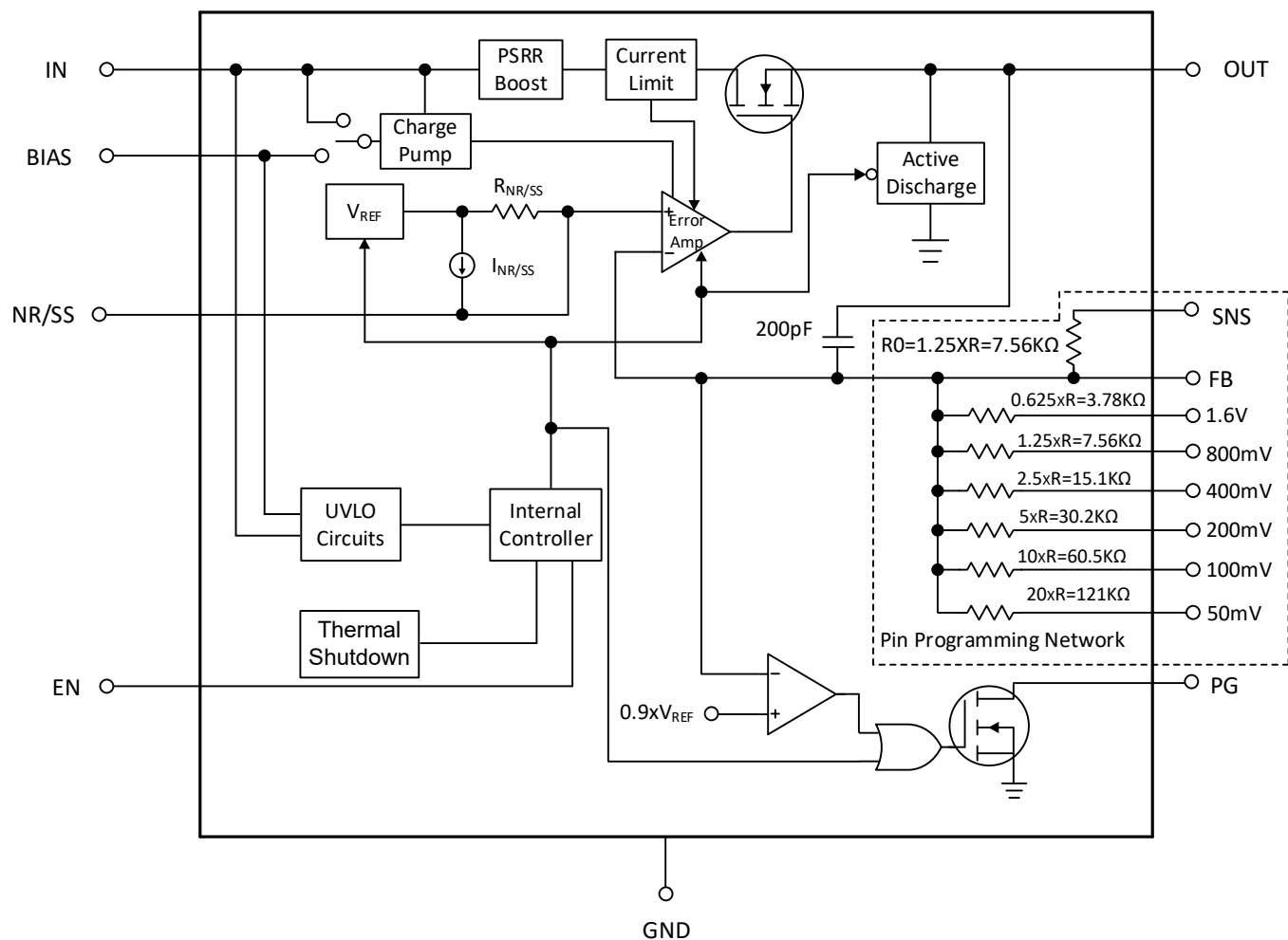
图 4. GM1203B-1 方框图
