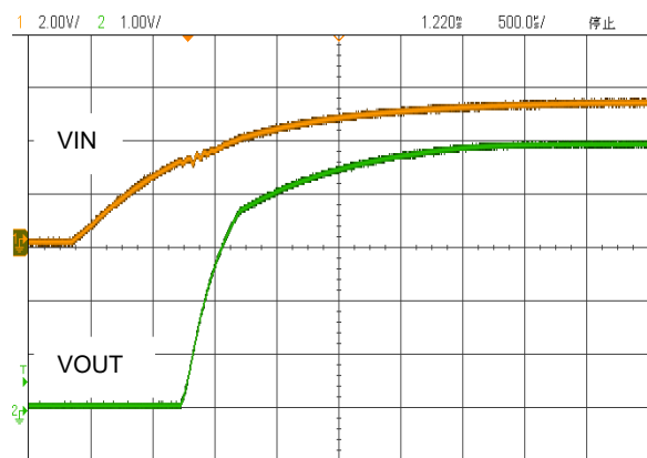
图 24. 软启动, V_{IN} = 5.3V , V_{OUT} = 5.0V , I_O = 3A
