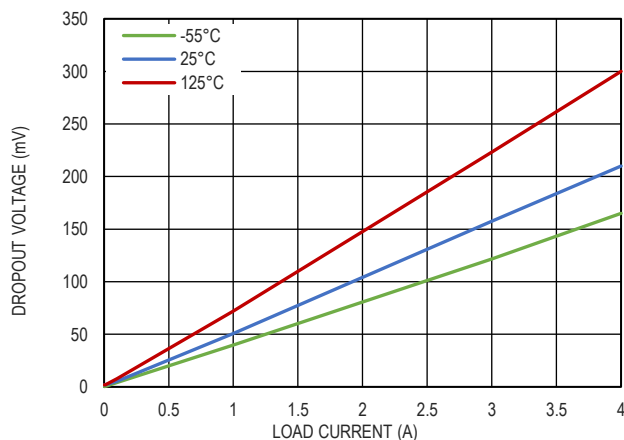
图 11. 压差电压和负载的关系, V_{OUT} = 1.5V , BIAS 浮空
