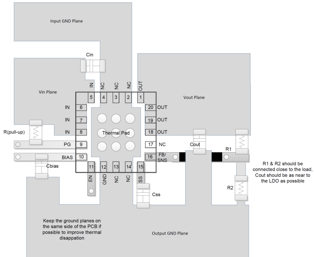
图 35. GM1203-2 布局示例
