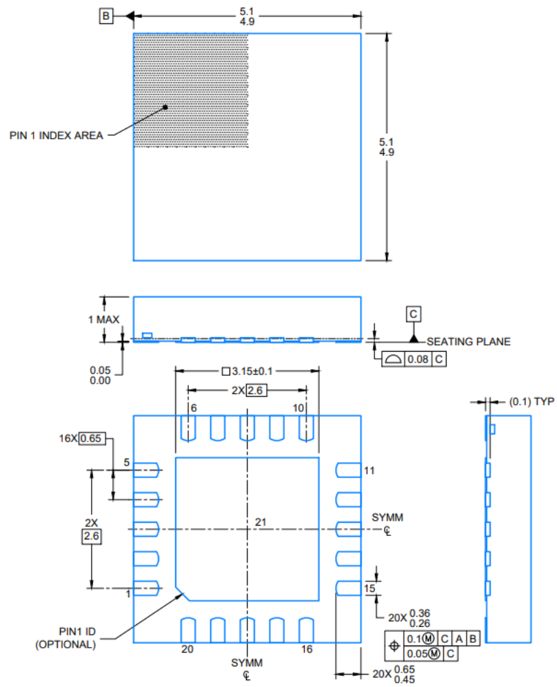
图 37. 20 引脚 QFN（5 毫米 x 5 毫米）
