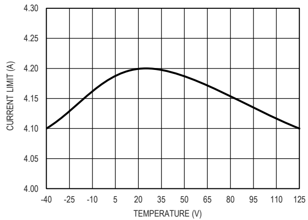
图 18. 输出限流值和温度的关系
