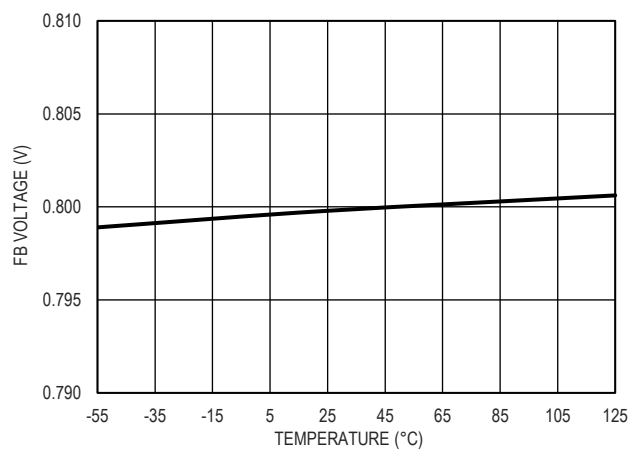
图 26. FB 引脚电压和温度的关系
