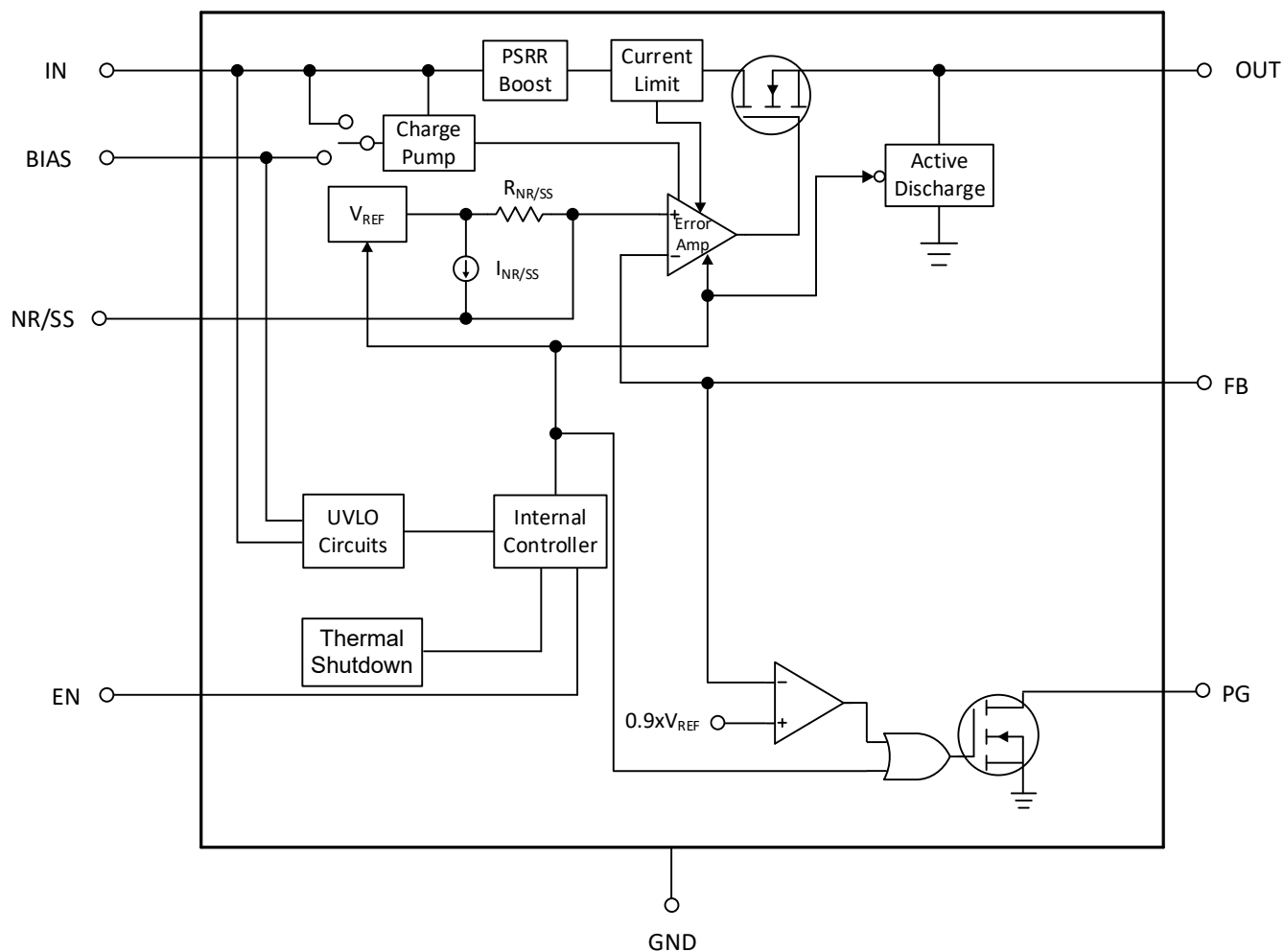
图 5. GM1203A-2 和 GM1203B-2 方框图
