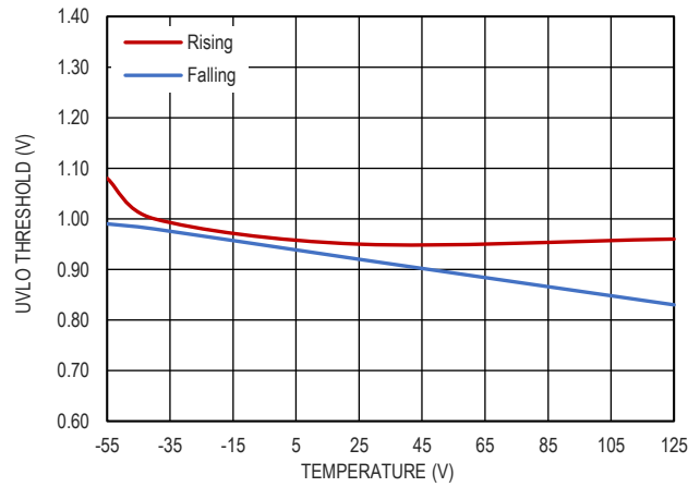
图 17. UVLO 阈值, V_{BIAS} = 5V
