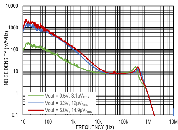
图 23. 输出噪声谱密度, V_{IN}=5V , V_{OUT}=3.3V
