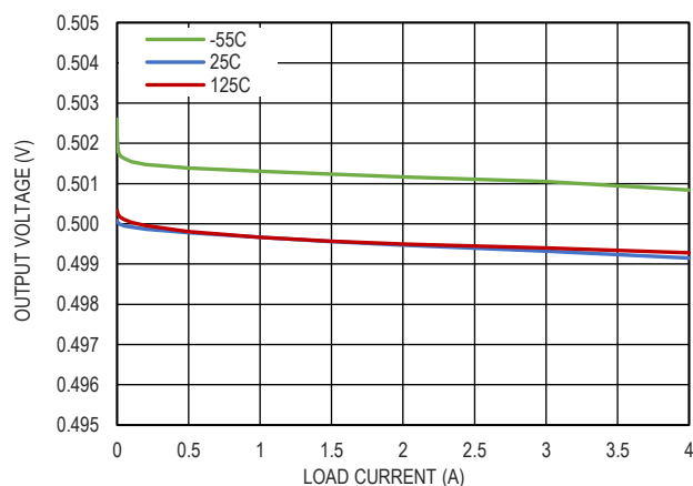
图 9. 负载调整率, BIAS 浮空
