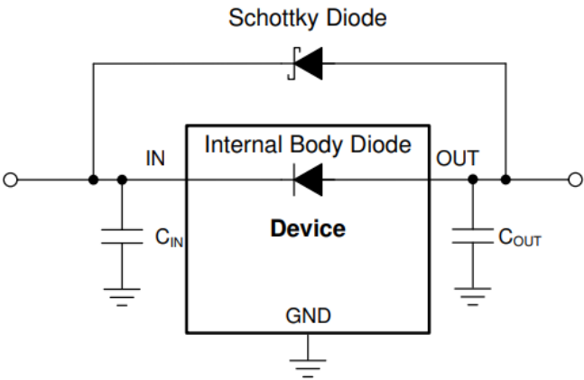
图 33. 反向电流保护应用电路
