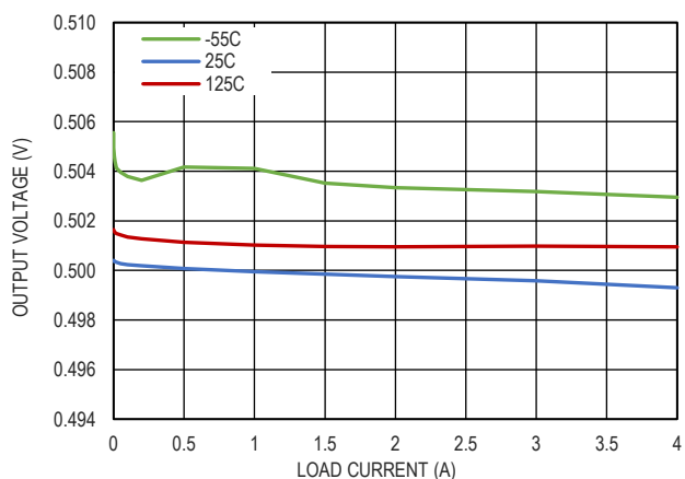
图 10. 负载调整率, V_{BIAS} = 5V
