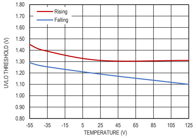
图 16. UVLO 阈值, BIAS 浮空
