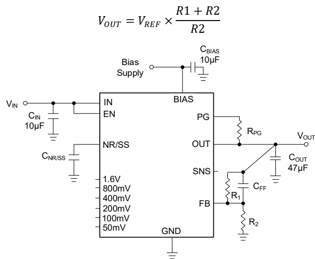
图 29 由外部电阻决定的输出电压
