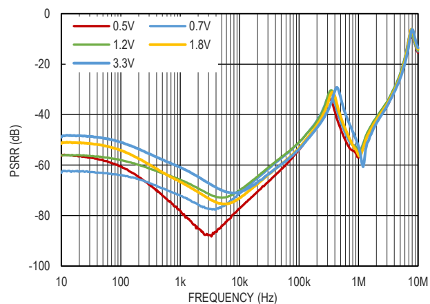
图 22. PSRR, V_{IN} = V_{OUT} + 0.4V , I_O = 3A
