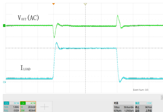
图 25. 负载跳变, V_{IN} = 2.8V , V_{OUT} = 1.8V , I_O = 0.3A 至 3A
