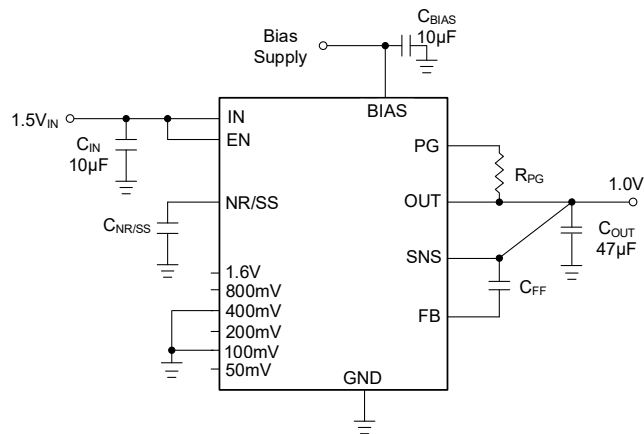
图 30 无需外部电阻的输出电压设置
