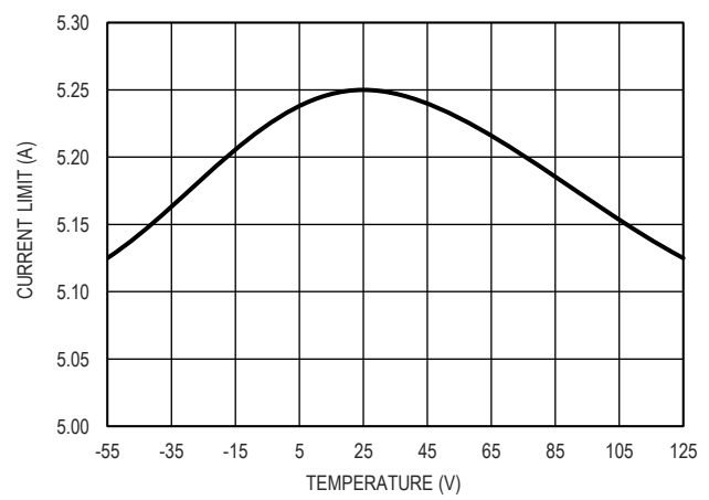
图 19. GM1203-3 输出限流值和温度的关系
