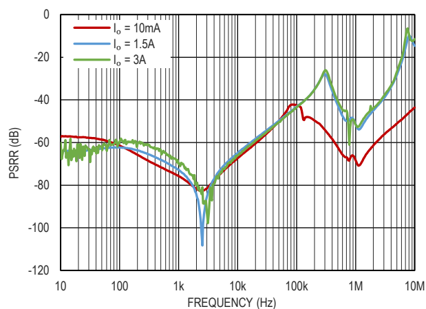
图 20. PSRR, V_{IN} = 1.1V , V_{OUT} = 0.8V , V_{BIAS} = 5.0V
