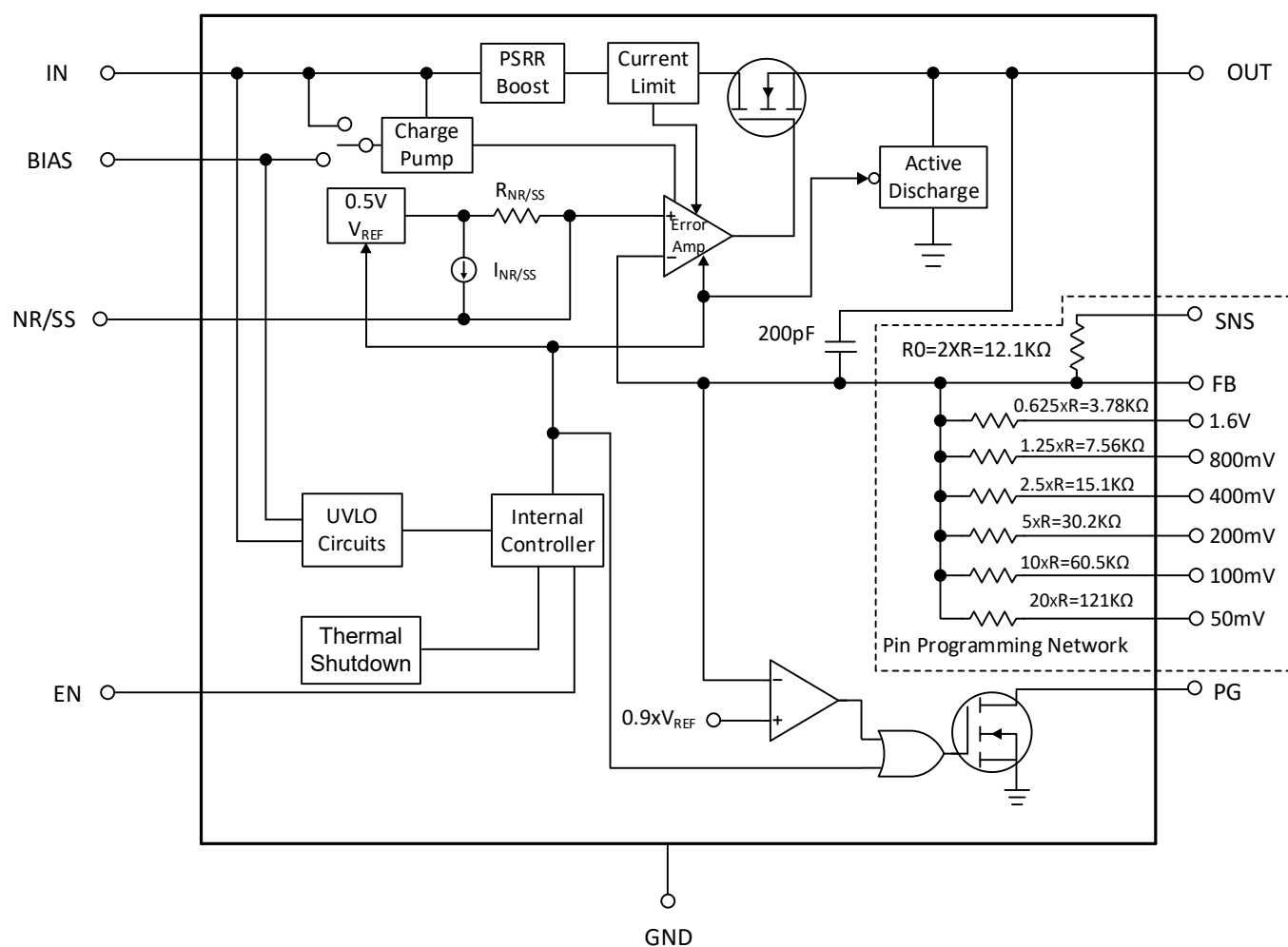
图 3. GM1203A-1 方框图
