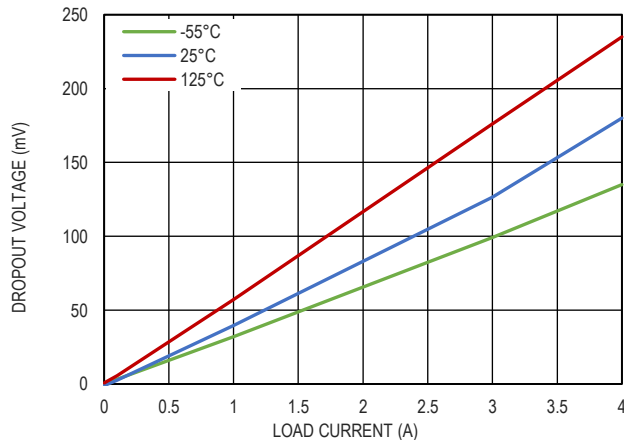
图 13. 压差电压和负载的关系, V_{OUT} = 1.2V , V_{BIAS} = 5V
