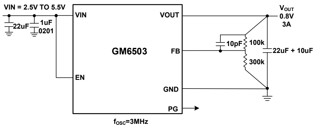
图 17. V_{IN}=3.3\text{V} , V_{OUT}=0.8\text{V} , I_{LOAD}=3\text{A}
