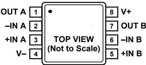
图 4.MSOP-8 和 SO-8 引脚配置(顶视图)
