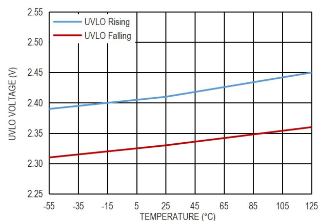
图 13. UVLO 阈值
