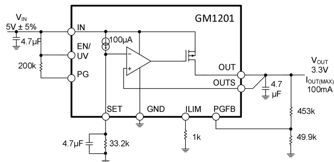
图 1 典型应用
