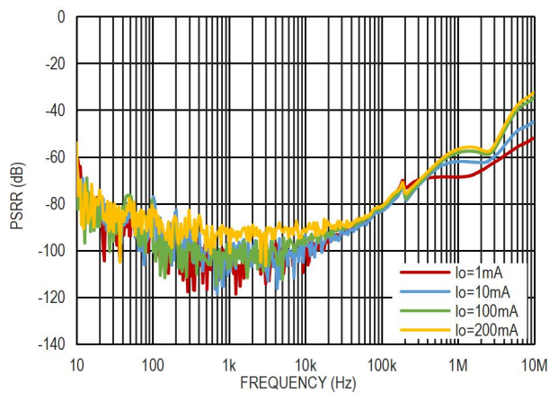
图 19. 电源电压纹波抑制比, V_{IN}=4.3V , V_{OUT}=3.3V
