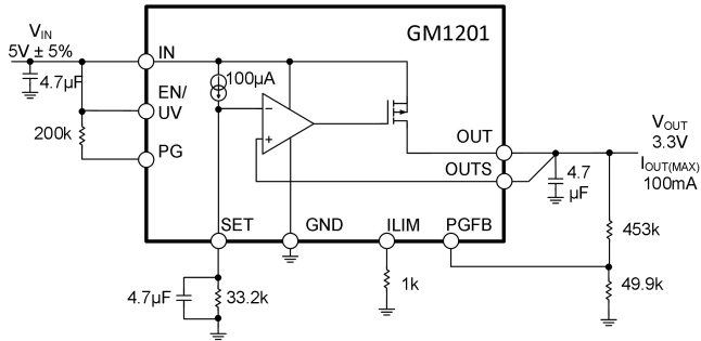
图 22 典型应用
