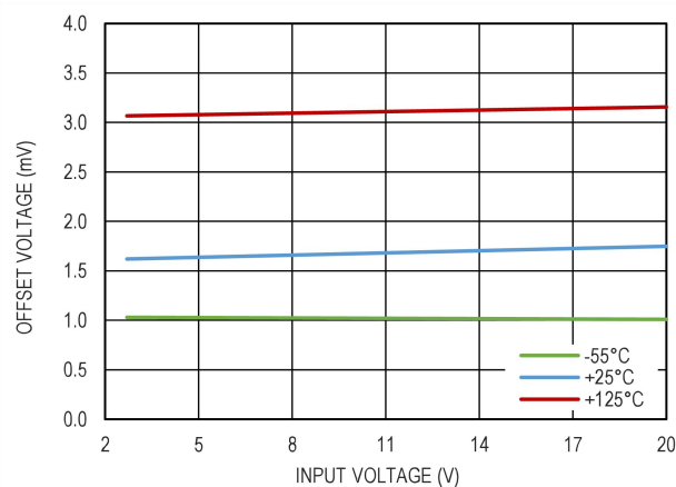
图 6. |V_{OUT}-V_{SET}| 和输入电压的关系, V_{OUT}=3.0V
