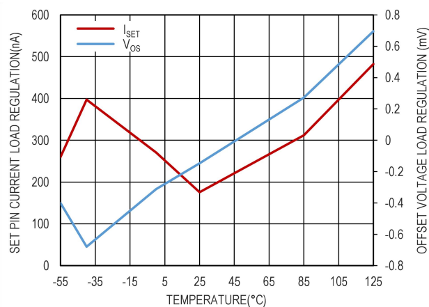
图 8. SET pin 电流、 |V_{OUT}-V_{SET}| 和温度的关系
