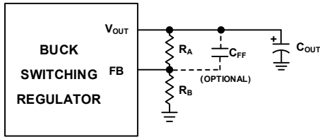
图 30. 反馈电阻网络
