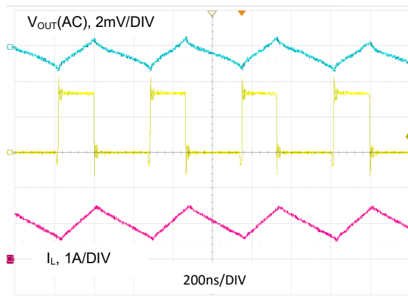
图 24. V_{OUT} = 1.2V , I_O = 1A , FPWM
