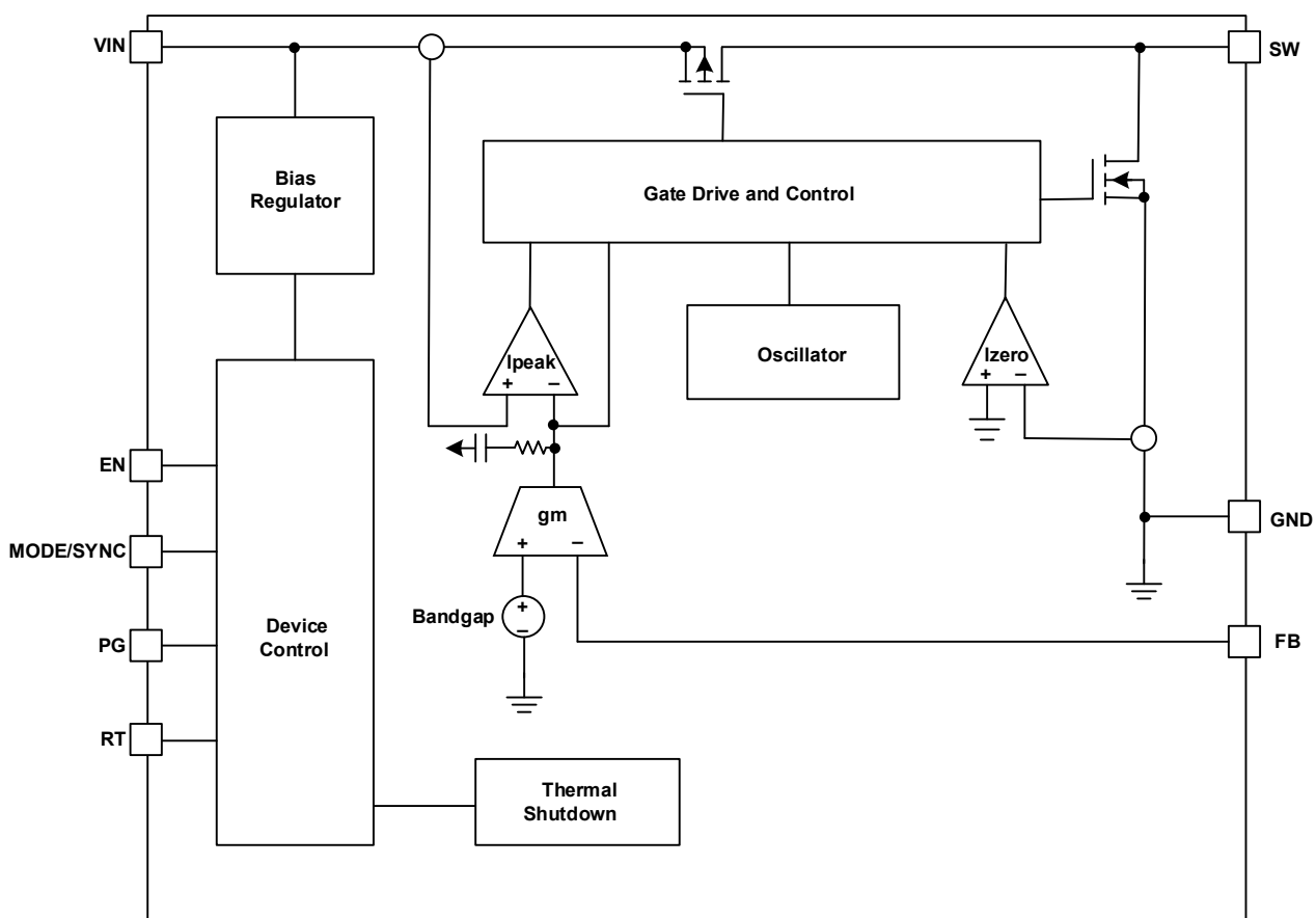
图 3 GM2500 功能框图
