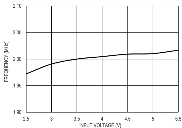
图 15. 频率和输入电压的关系, RT 接高
