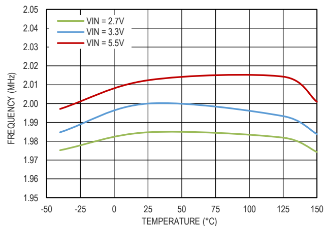
图 17. 频率和温度的关系, RT 接高
