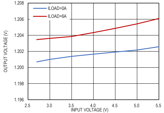
图 19. 输出电压线调整率, V_{OUT} = 1.2V
