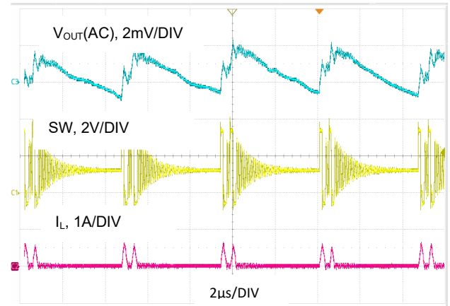
图 25. V_{OUT} = 1.2V , I_O = 100mA , PSM 模式
