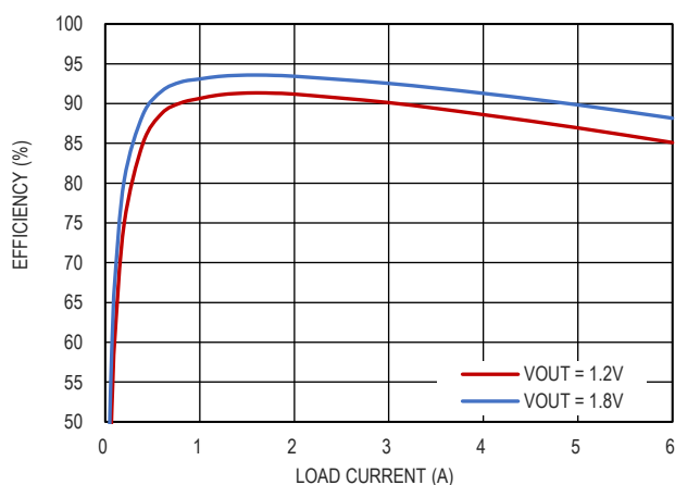
图 12. 效率曲线, V_{IN} = 3.3V , F_{SW} = 4MHz , FPWM
