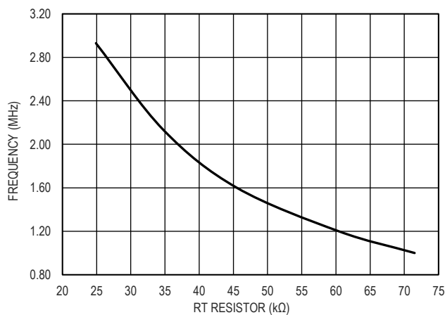
图 16. 频率和 RT 电阻的关系
