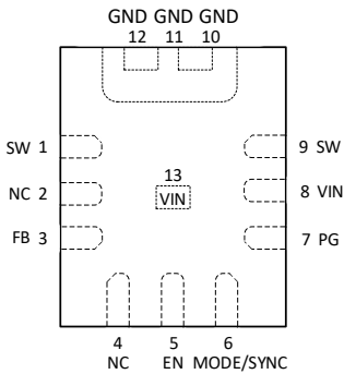
13 引脚 LQFN (2mm x 3mm) 图 5 引脚配置
