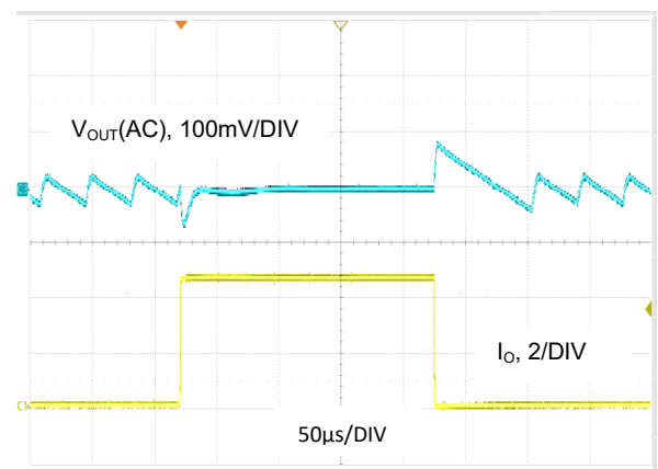
图 29. V_{OUT} = 1.2V , I_O = 0.1A 至 4.5A , 低功耗模式
