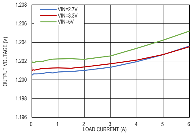
图 18. 输出电压负载调整率, V_{OUT} = 1.2V
