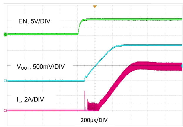
图 23. 启动波形, V_{OUT} = 1.2V , I_O = 6A
