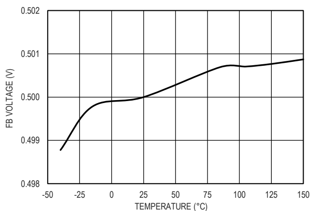
图 14. FB 引脚电压和温度的关系
