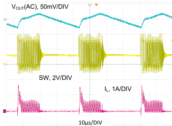
图 26. V_{OUT} = 1.2V , I_O = 10mA , 低功耗模式
