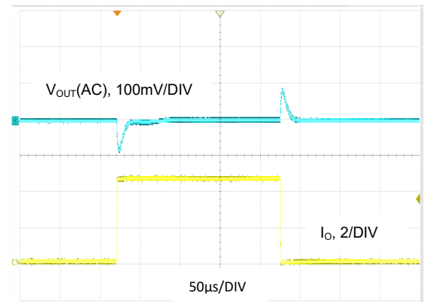
图 27. V_{OUT} = 1.2V , I_O = 0.1A 至 4.5A , FPWM 模式
