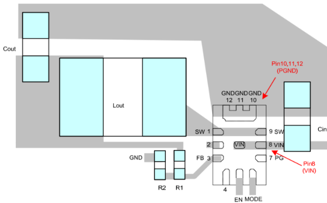
图 32. GM25002 PCB 推荐布局
