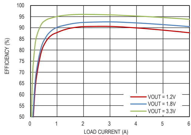
图 13. 效率曲线, V_{IN} = 5V , F_{SW} = 4MHz , FPWM
