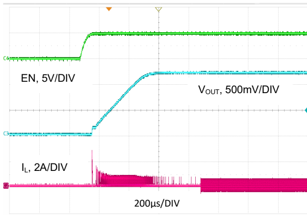
图 22. 启动波形, V_{OUT} = 1.2V , I_O = 10mA
