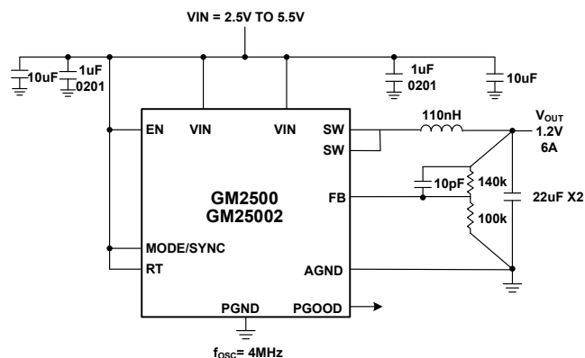
图 2. 4MHz 典型应用
