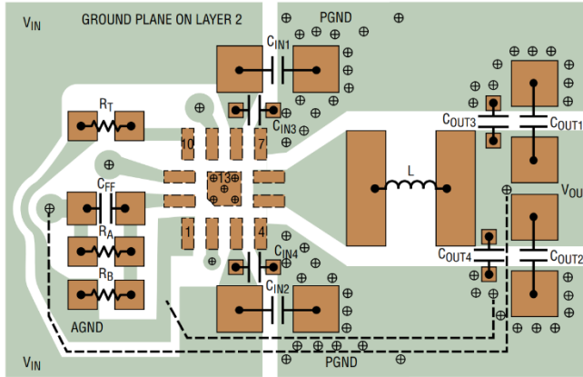
图 31. GM2500 和 GM25001 PCB 推荐布局
