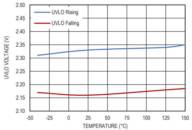
图 21. UVLO 阈值和温度的关系
