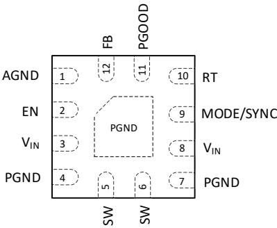
12 引脚 LQFN (2mm x 2mm) 图 4 引脚配置
