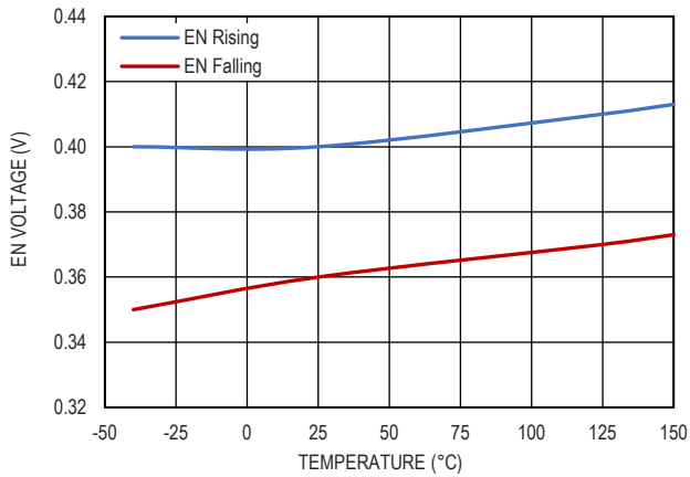
图 20. EN 阈值和温度的关系
