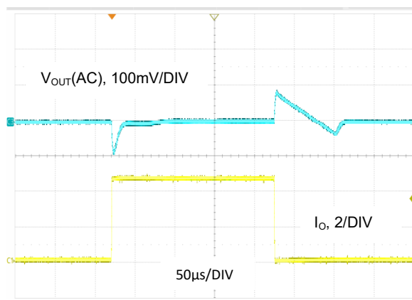
图 28. V_{OUT} = 1.2V , I_O = 0.1A 至 4.5A , PSM 模式
