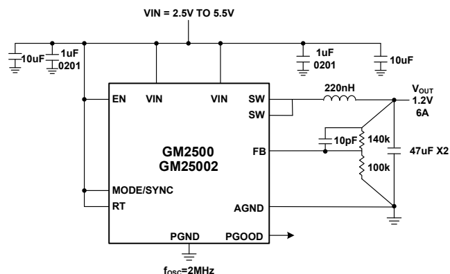
图 1. 2MHz 典型应用
