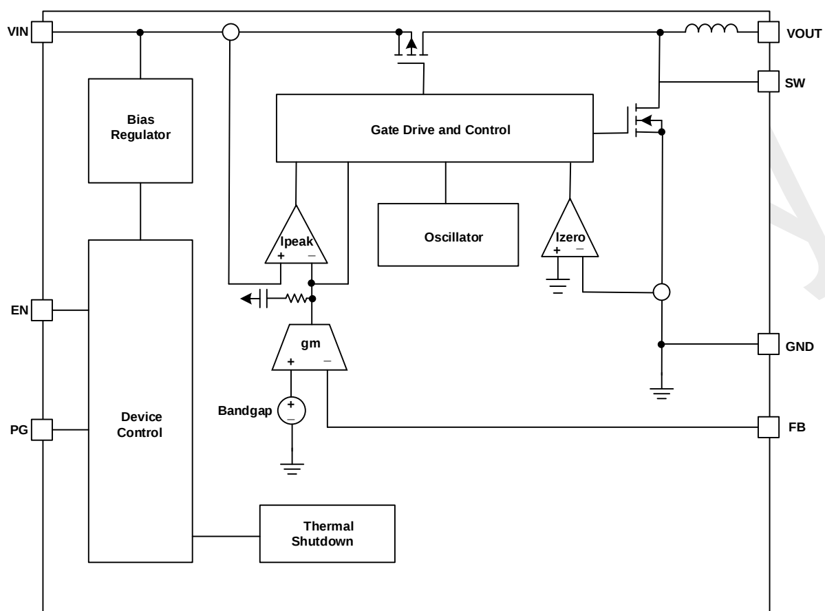
图 2 GM6503A 功能框图
