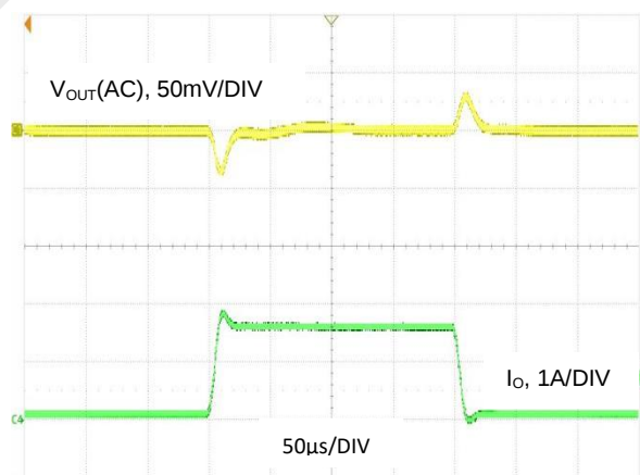
图 15. V_{OUT} = 1.2\text{V} , I_o = 0.1\text{A} 至 1.6\text{A} , FPWM 模式
