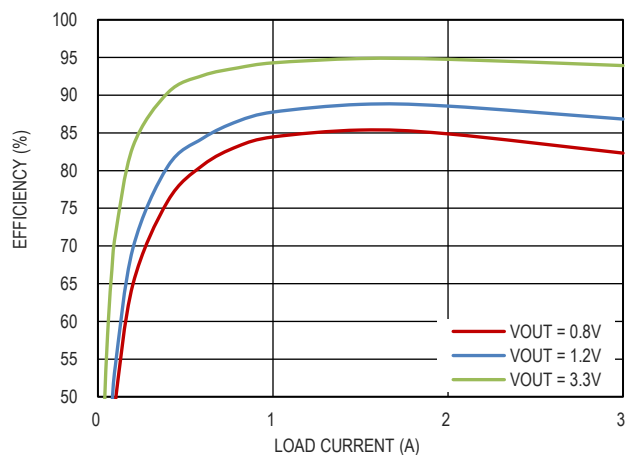
图 5. 效率曲线, V_{IN} = 5V
