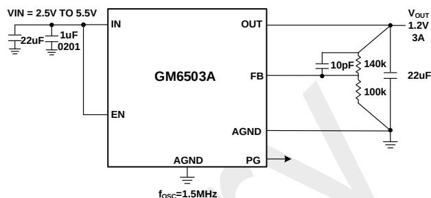
图 1. GM6503A 典型应用
