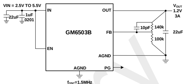
图 1. GM6503B 典型应用
