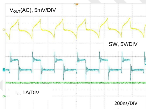
图 14. V_{OUT} = 1.2\text{V} , I_o = 1\text{A} , FPWM 模式
