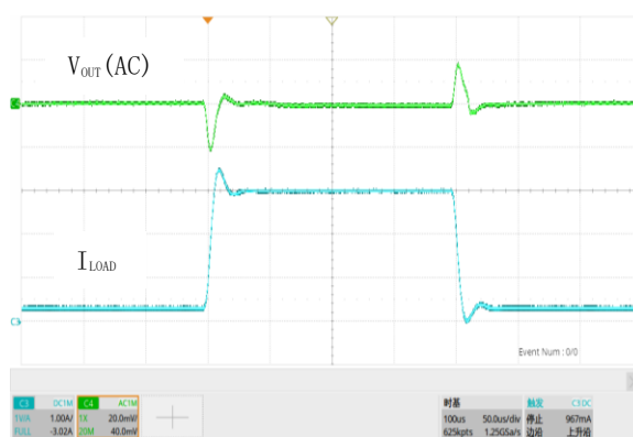
图 19. 负载瞬态响应, V_{IN}=2.8V , V_{OUT}=1.8V , I_{OUT}=0.1A to 1.5A
