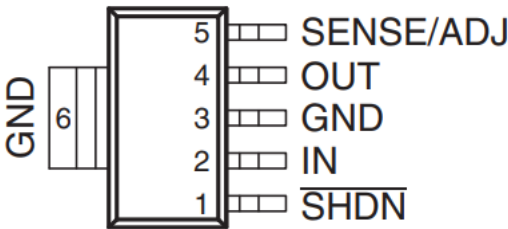
5 引脚 SOT-223 裸露焊盘必须焊接到 PCB 上
