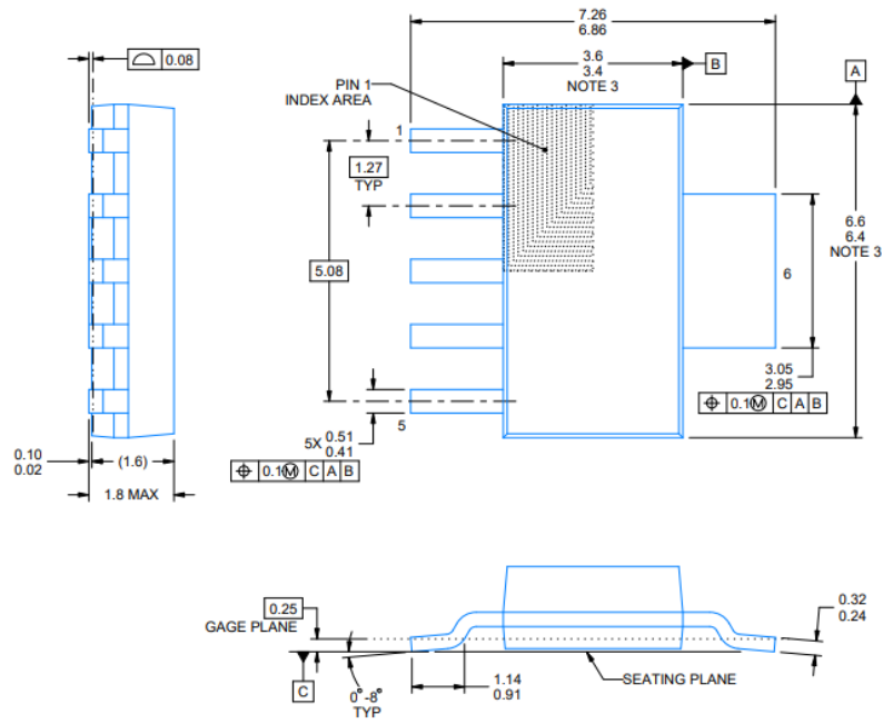
图 22.5 引脚 SOT-223
