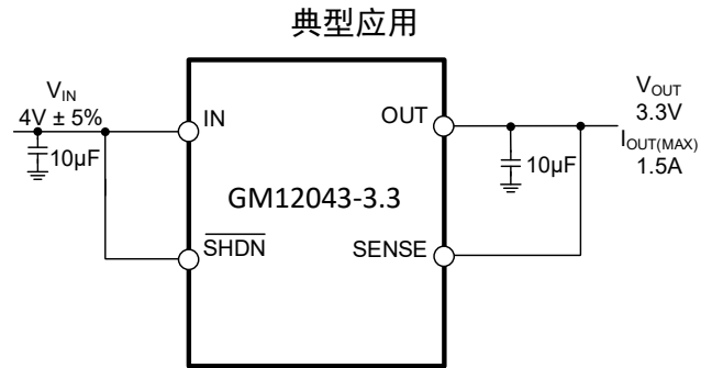
图 1 典型应用
