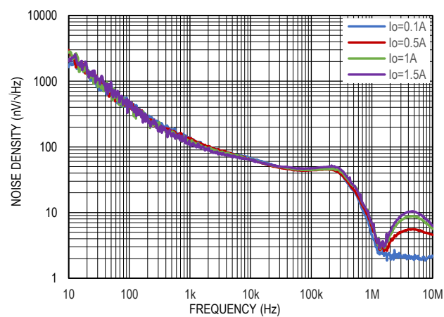
图 15. 输出噪声谱密度, V_{IN}=5V , V_{OUT}=3.3V
