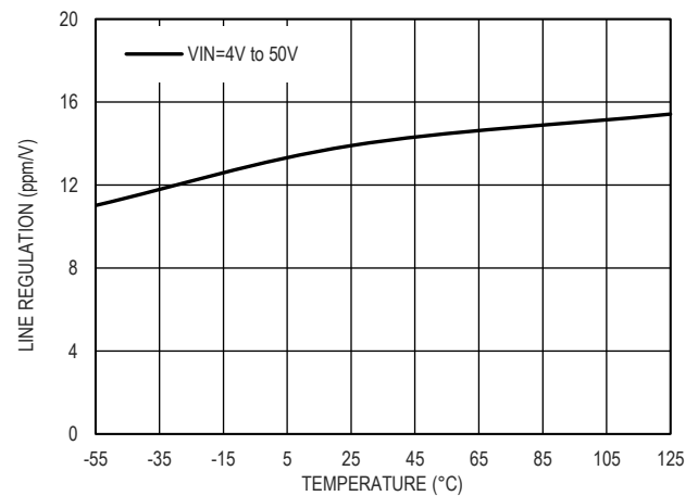
图 14. 输入调整率和温度的关系, V_{OUT}=2.048V
