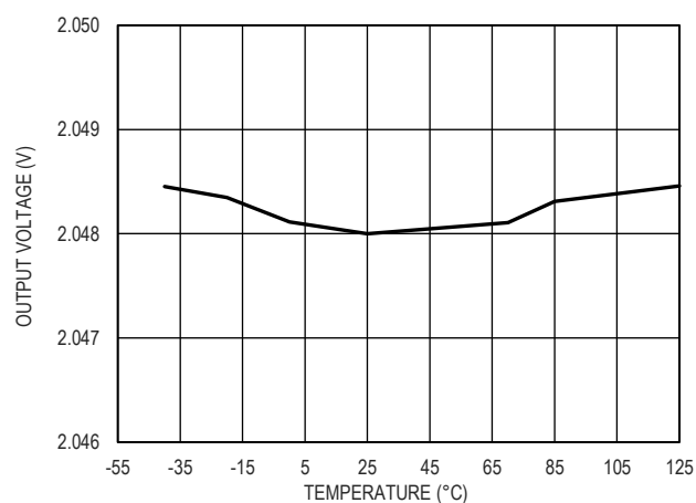
图 6. 2.048V 输出电压和温度的关系
