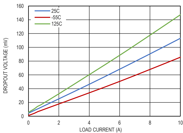
图 21. 最小输入电压和输出电压的关系, V_{OUT}=3.3V
