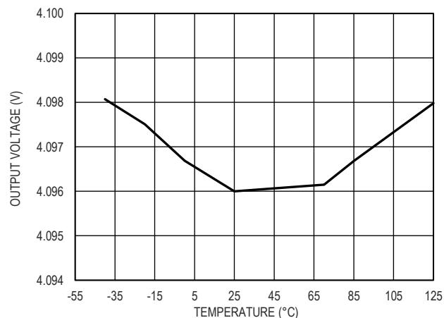
图 8. 4.096V 输出电压和温度的关系
