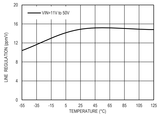
图 16. 输入调整率和温度的关系, V_{OUT}=4.096V
