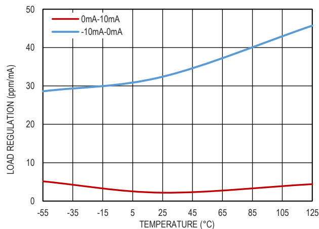
图 10. 负载调整率和温度的关系, V_{OUT}=2.048V
