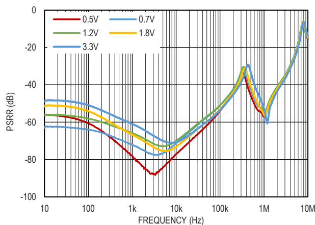
图 22. PSRR, V_{IN} = V_{OUT} + 0.4V , I_O = 3A
