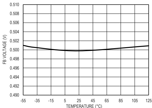
图 8. FB 引脚电压和温度的关系
