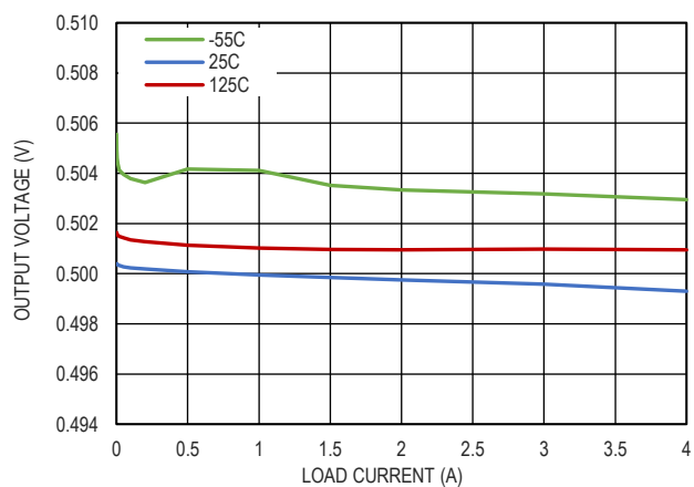
图 10. 负载调整率, V_{BIAS} = 5V
