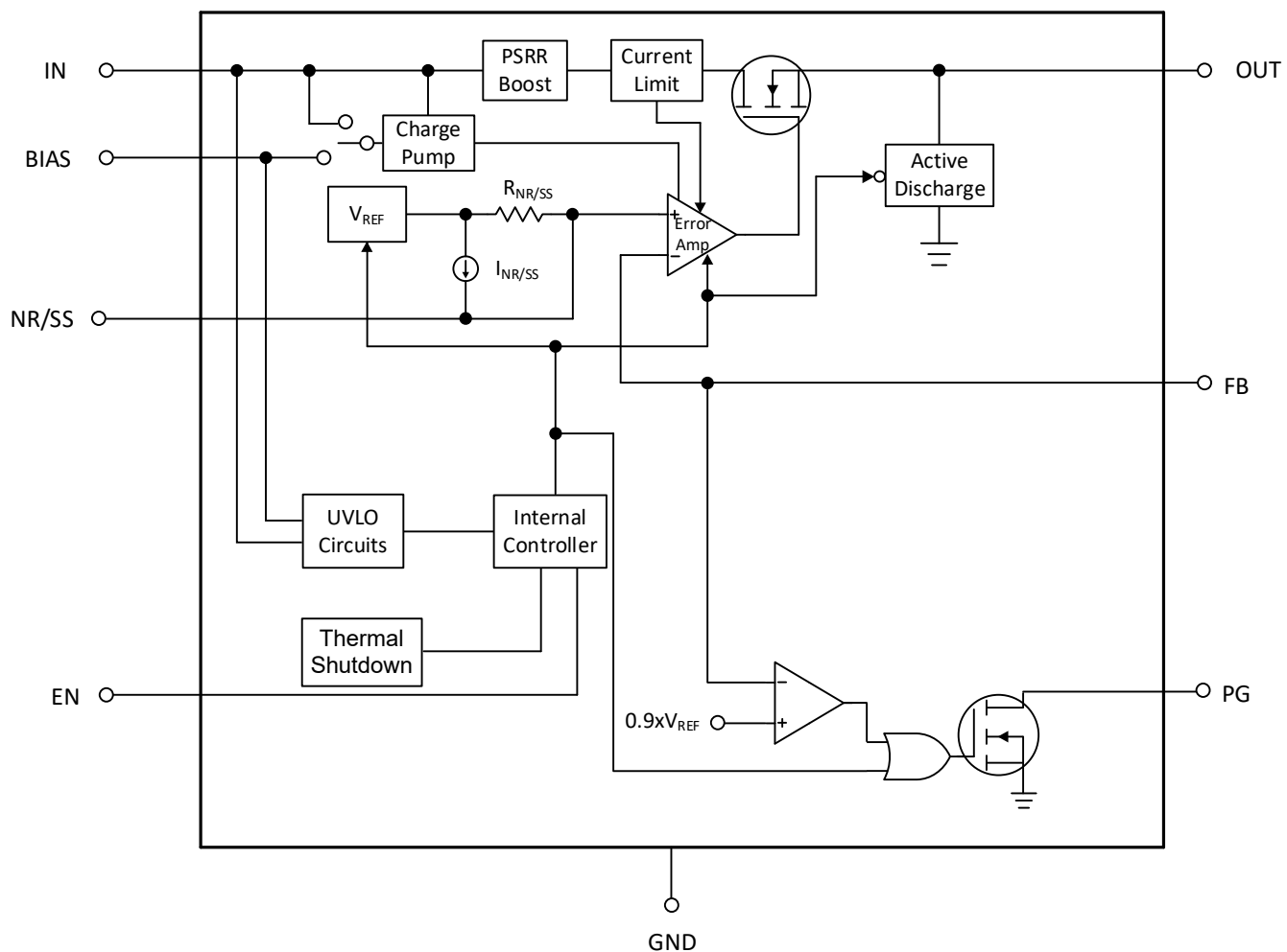
图 5. GM1203A-2 和 GM1203B-2 方框图
