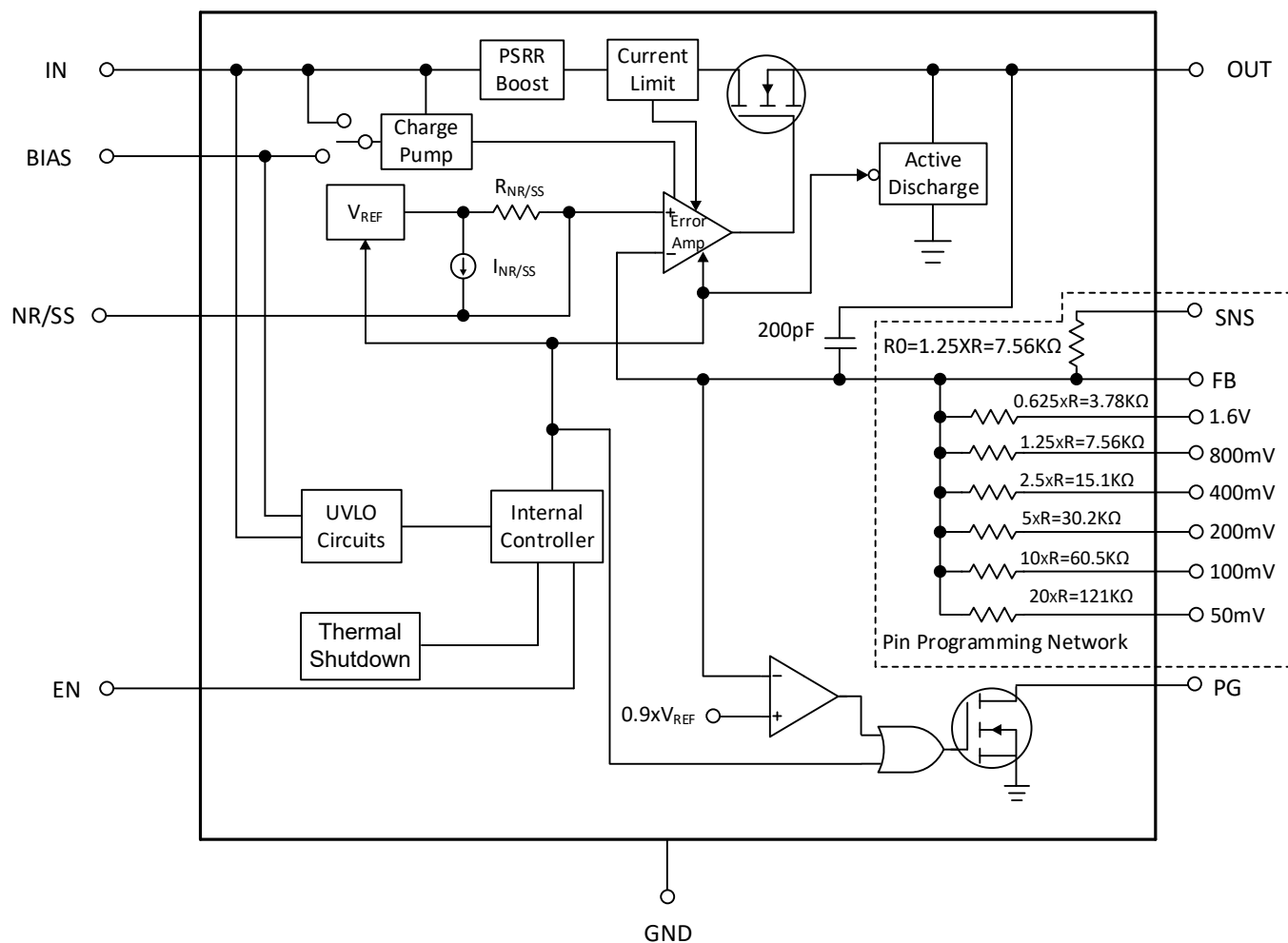
图 4. GM1203B-1 方框图
