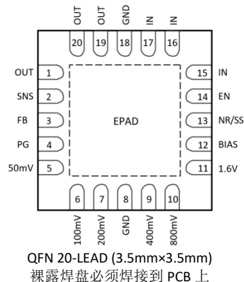
图 6 引脚配置
