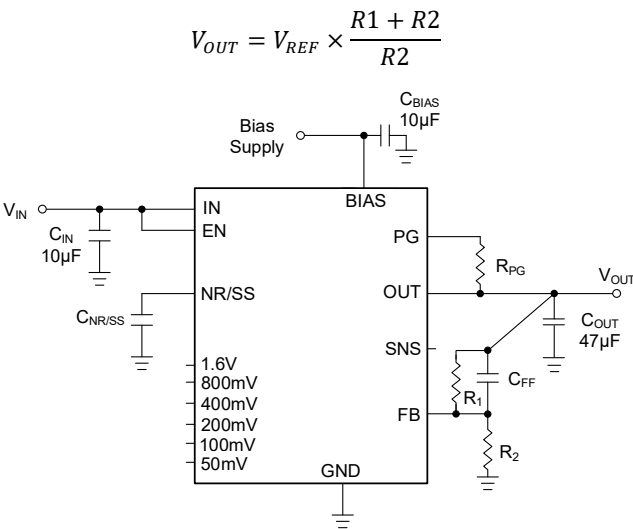
图 29 由外部电阻决定的输出电压
