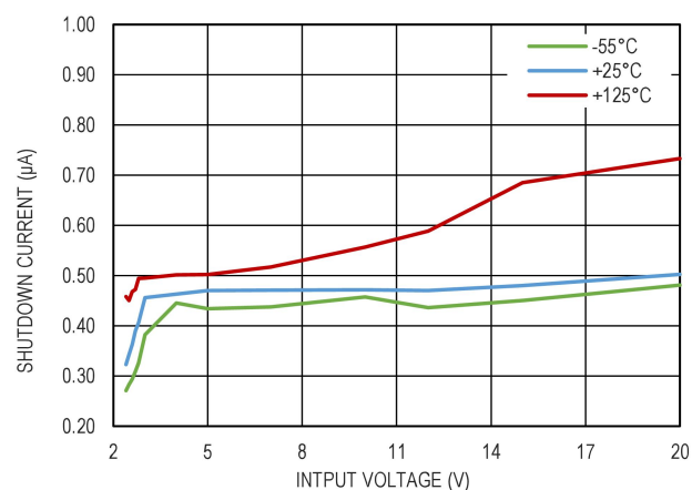
图 11. 停机静态电流和输入电压的关系
