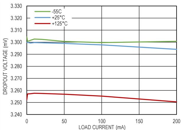
图 9. V_{OUT} = 3.3V 时的负载调整率
