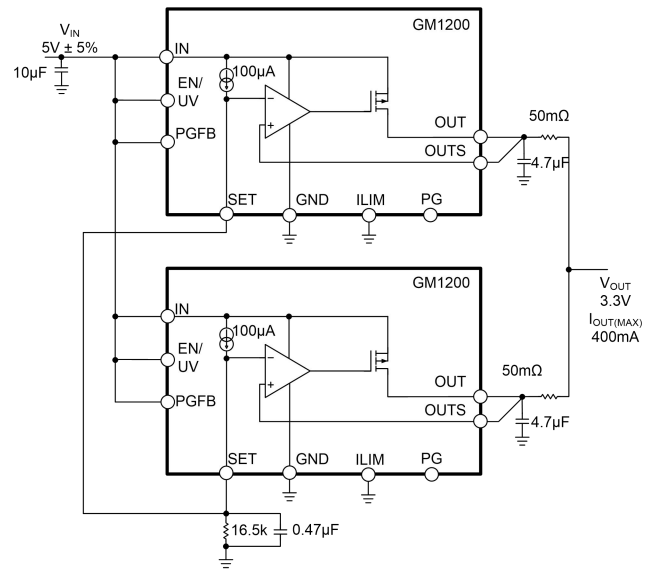
图 23 并联设备
