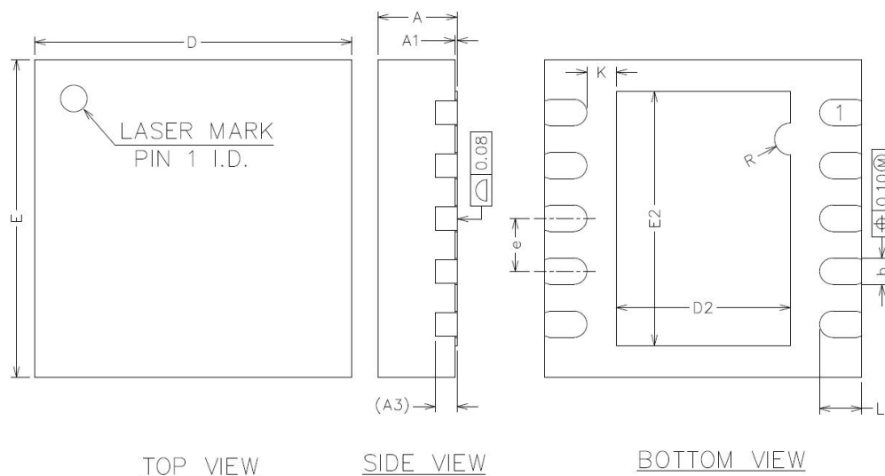
图 24 DFN 封装 (3mmx3mm)
