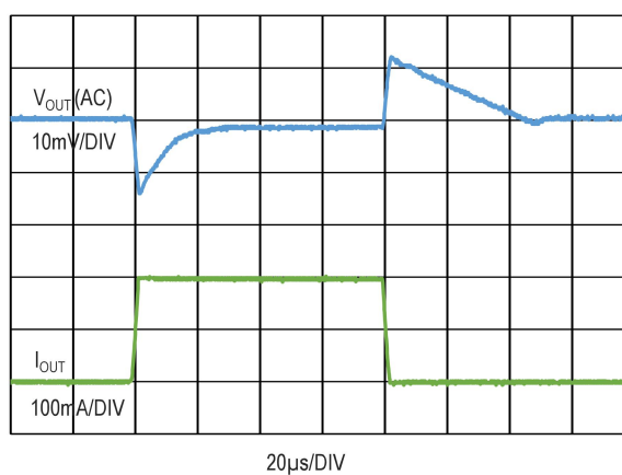
图 21. 负载瞬态响应, V_{IN}=4V , V_{OUT}=3.3V , I_{OUT}=1mA to 200mA
