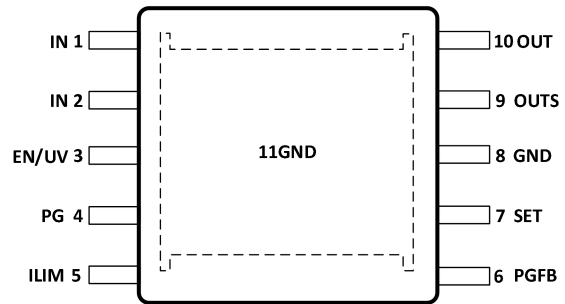
图 3. MSOP 引脚配置(顶视图)
