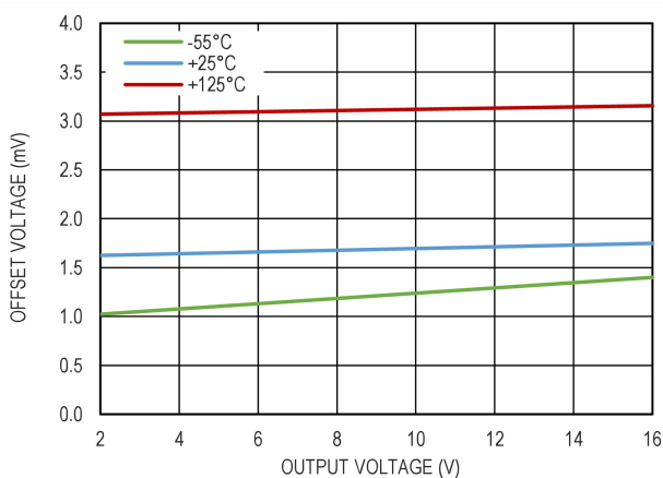
图 7. |V_{OUT} - V_{SET}| 和输出电压的关系
