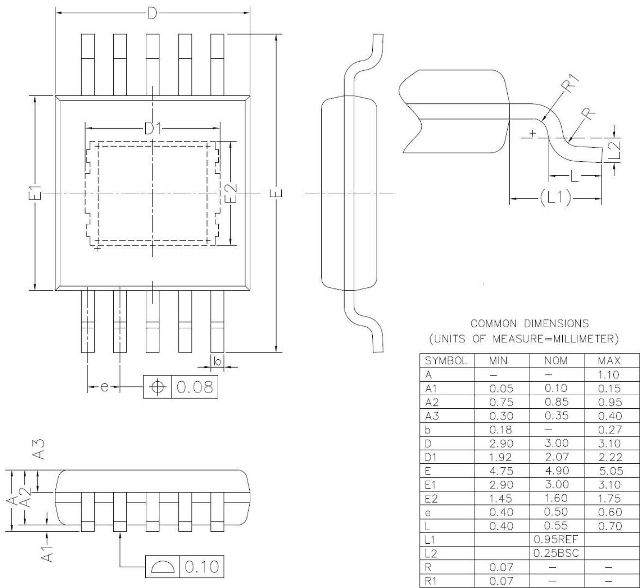
图 25 MSOP 封装
