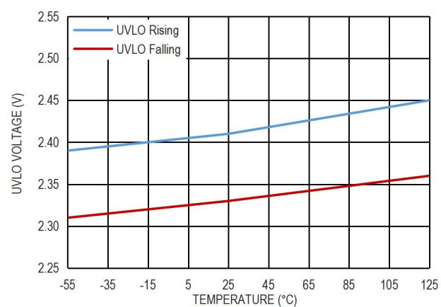
图 13. UVLO 阈值
