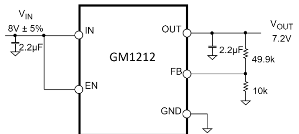
图 2. 可调输出至 7.2V
