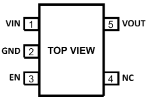
图 5.5 引脚 SOT-23 引脚配置（固定输出）
