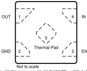
图 3.5 引脚 DFN-5 的引脚配置（固定输出）
