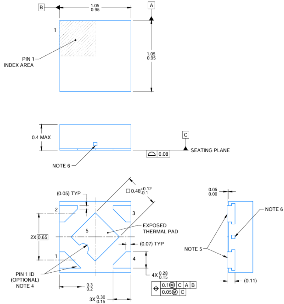
图 26.4 脚 DFN-4
