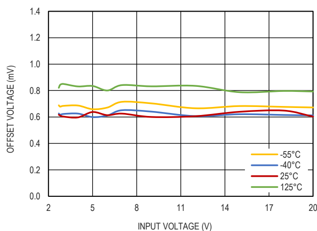
图 10. |V_{OUT}-V_{SET}| 和输入电压的关系, V_{OUT}=1.8V
