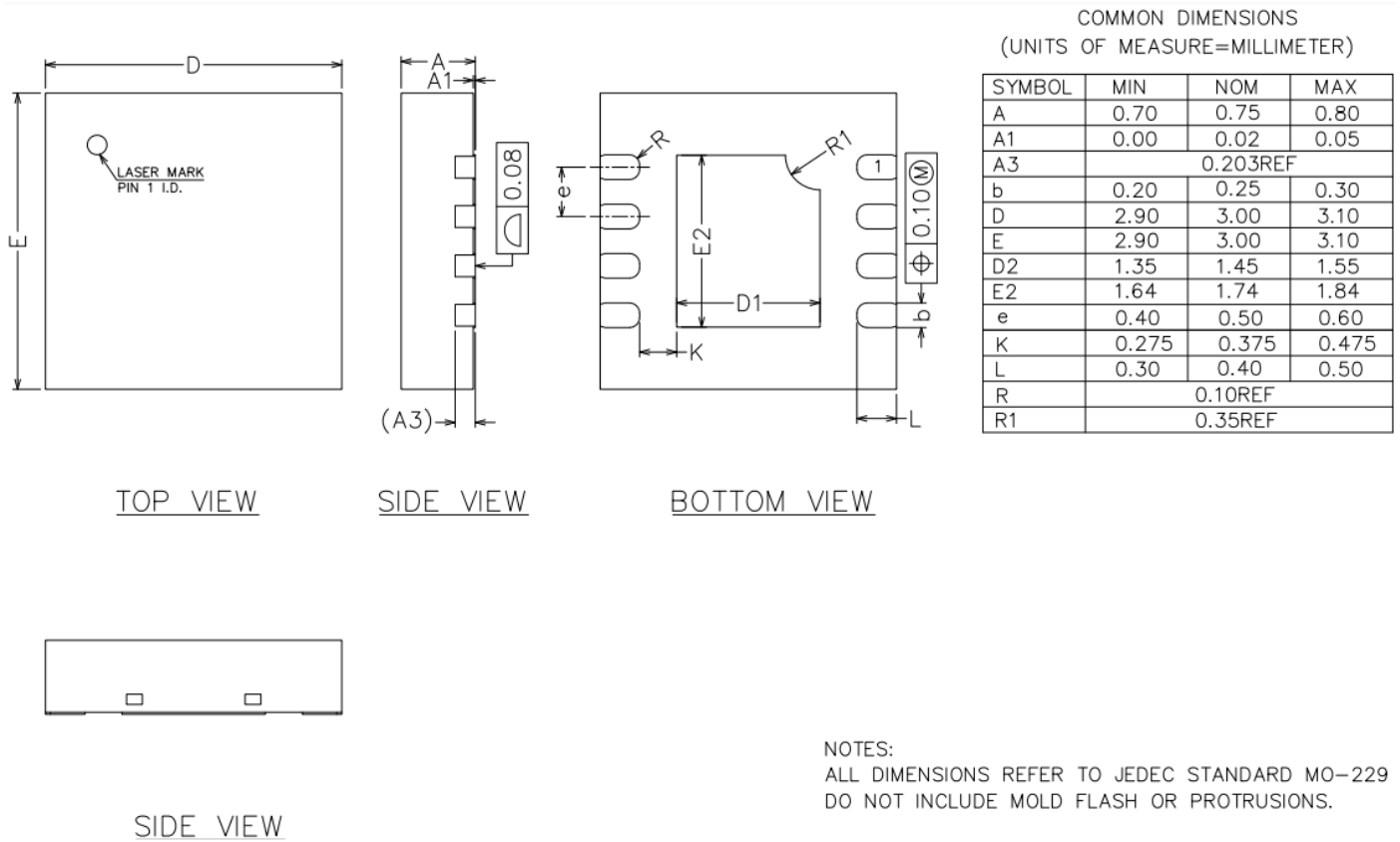
图 33. DFN-8 封装 (3mmx3mm)
