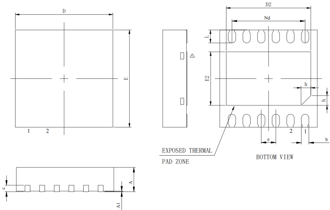
图 32. DFN12 封装 (3mmx3mm, CP-12-1)
