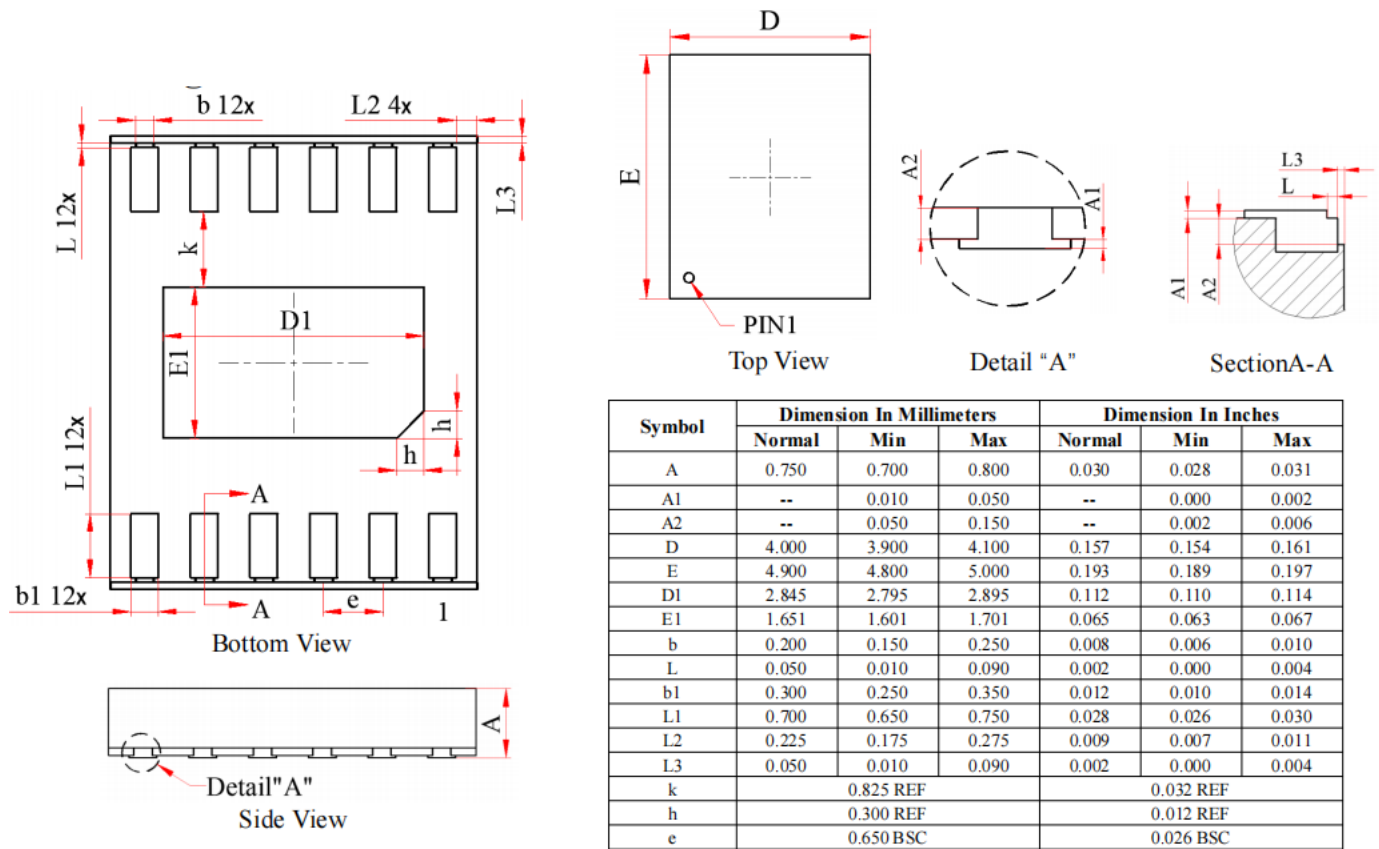
图 31. DFN12 封装 (4mmx4.9mm, CP-12-2) 和 MSOP-12 管脚兼容
