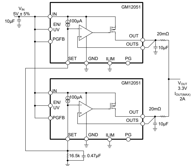
图 28. 并联设备
