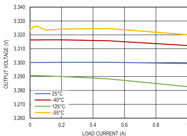
图 13. V_{OUT}=3.3V 时的负载调整率
