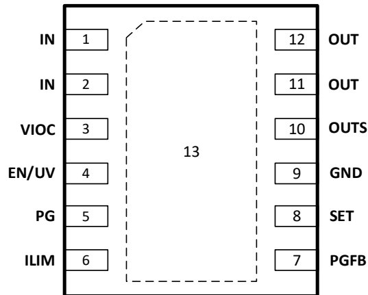
图 6. GM12051ACPZ-1 4mmx4.9mm DFN12 兼容 MSOP-12 和 GM12051ACPZ-2 3mmx3mm DFN12 引脚配置(顶视图)
