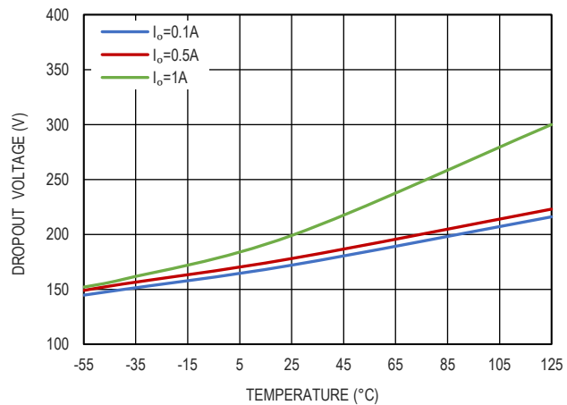
图 16. 压差电压和负载电流的关系, V_{OUT}=3.0V
