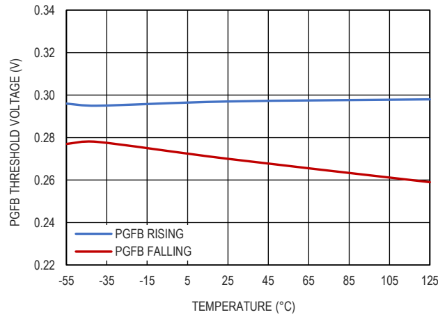
图 20. PGFB pin 阈值
