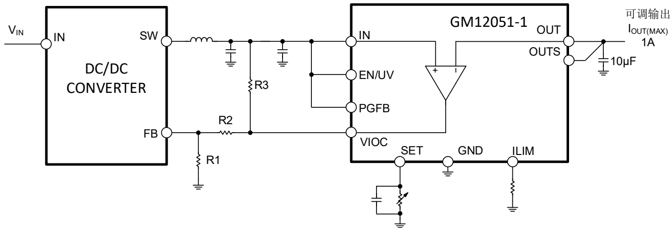
图 29. VIOC 典型应用
