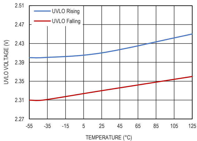
图 17. UVLO 阈值
