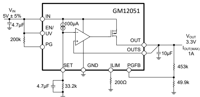
图 1 典型应用
