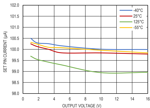
图 9. SET pin 电流和输出电压的关系
