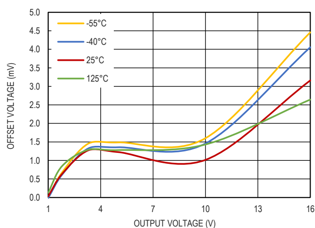
图 11. |V_{OUT}-V_{SET}| 和输出电压的关系
