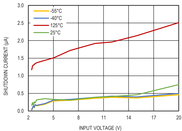
图 15. 停机静态电流和输入电压的关系
