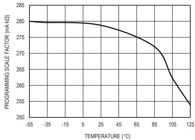
图 19. 输出限流值编程因子
