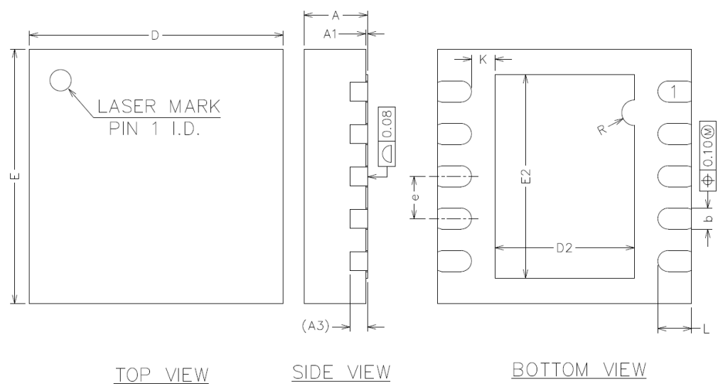
图 30. DFN-10 封装 (3mmx3mm)
