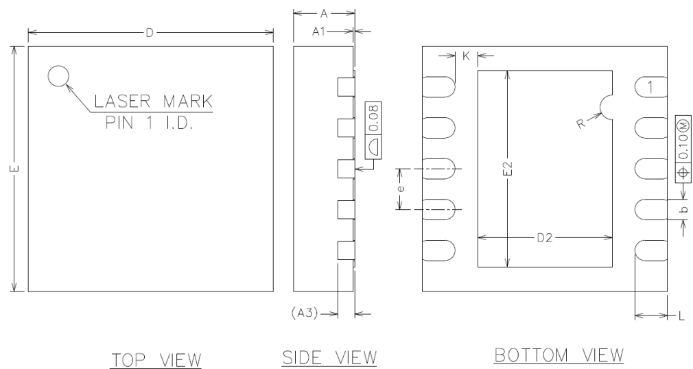
图 22. DFN10 封装 (3mmx3mm)
