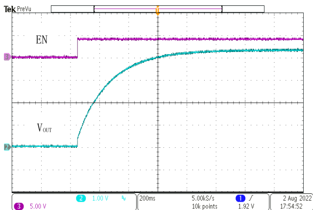
图 19. 软启动, V_{IN}=4.3V , V_{OUT}=3.3V , I_{OUT}=300mA
