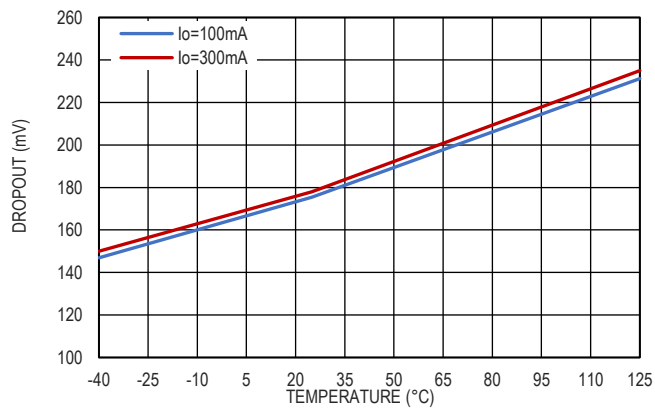
图 11. 压差电压和负载电流的关系, V_{OUT}=5.0V
