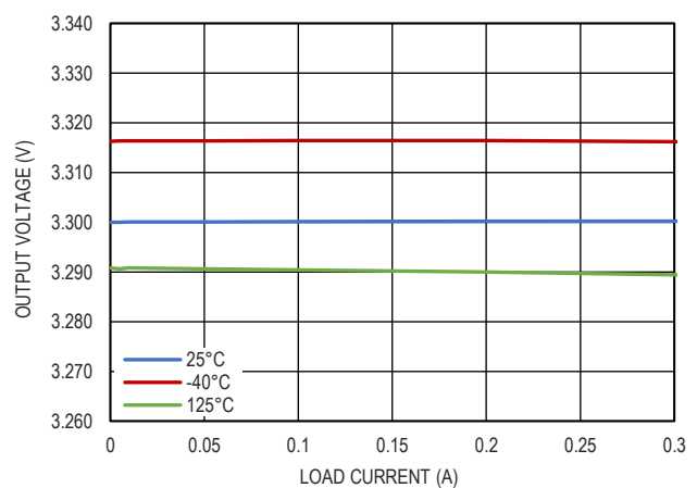
图 8. V_{OUT}=3.3V 时的负载调整率
