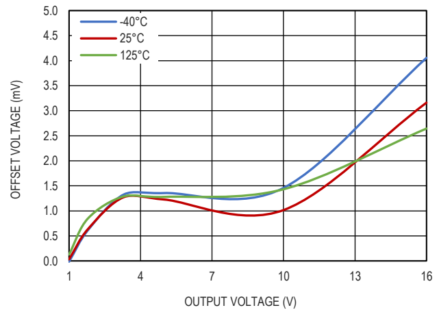
图 6. |V_{OUT}-V_{SET}| 和输出电压的关系
