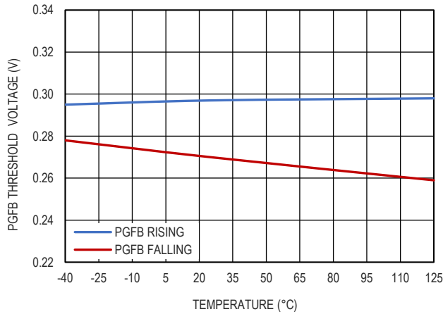
图 15. PGFB pin 阈值
