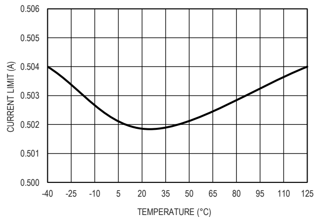
图 13. 输出限流值和温度的关系
