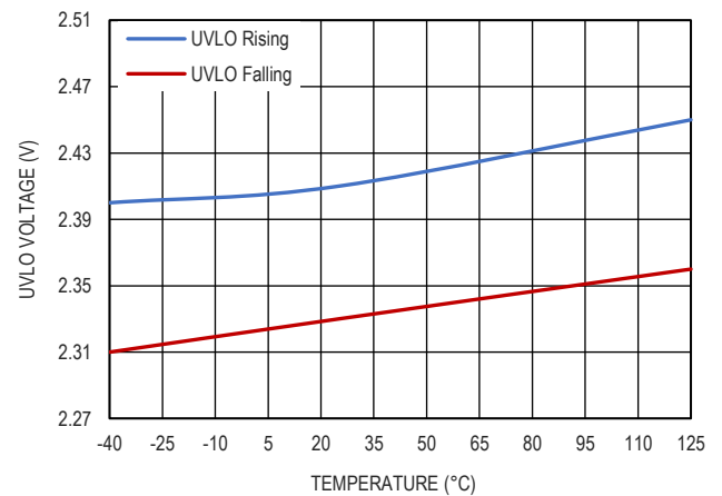
图 12. UVLO 阈值
