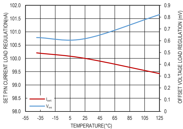
图 7. SET pin 电流温度的关系
