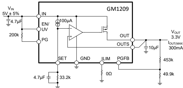
图 21 典型应用
