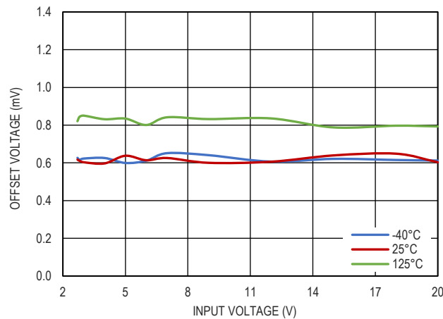
图 5. |V_{OUT}-V_{SET}| 和输入电压的关系, V_{OUT}=1.8V
