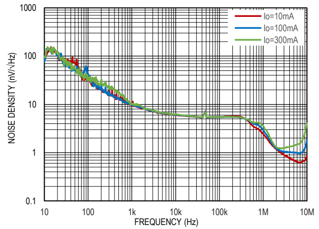
图 16. 输出噪声谱密度, V_{IN}=5V , V_{OUT}=3.3V
