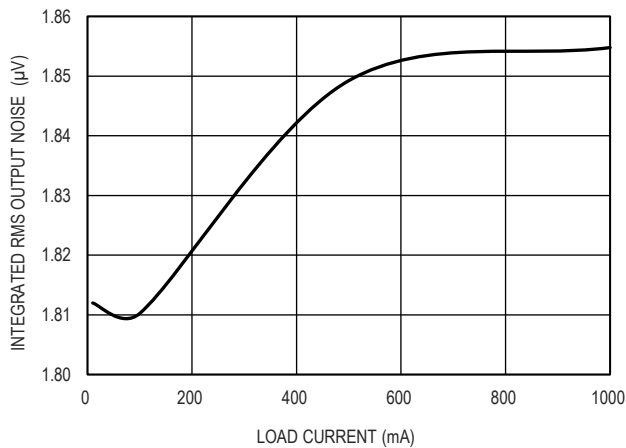
图 17. 积分 RMS 输出噪声, V_{IN}=5V , V_{OUT}=3.3V
