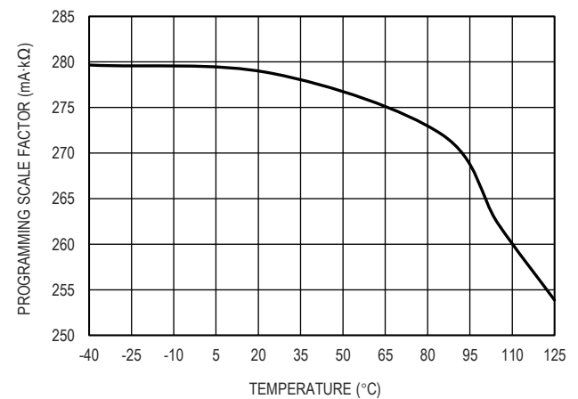
图 14. 输出限流值编程因子
