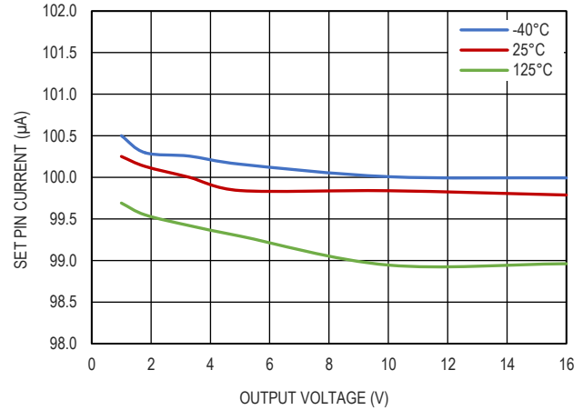
图 4. SET pin 电流和输出电压的关系
