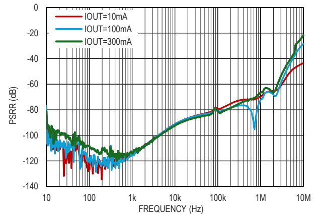
图 18. 电源电压纹波抑制比, V_{IN}=5V , V_{OUT}=3.3V
