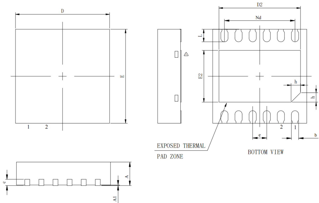
图 28. GM1205ACPZ-2-R7 DFN12 封装 (3mmx3mm, CP-12-1)
