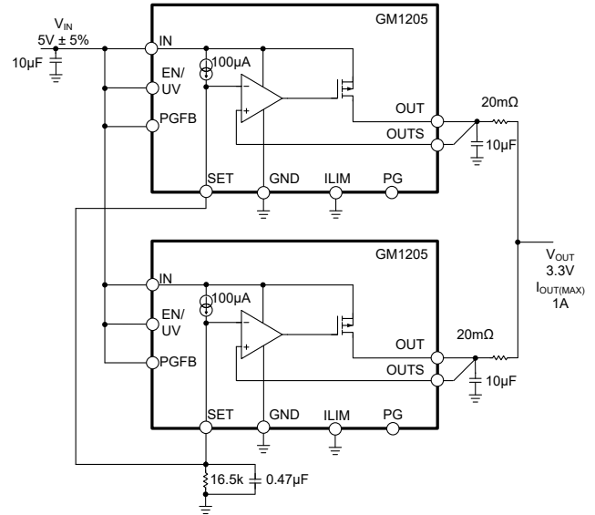
图 24. 并联设备
