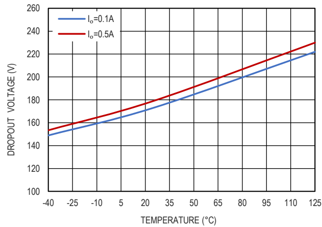
图 13. 压差电压和负载电流的关系, V_{OUT}=3.0\text{V}
