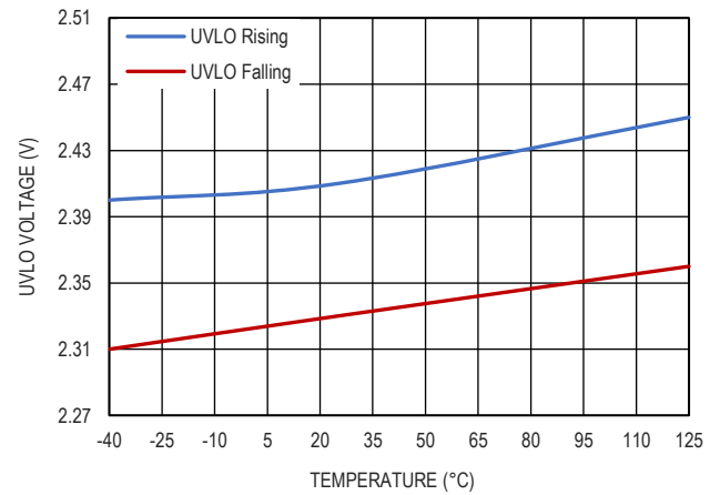
图 14. UVLO 阈值
