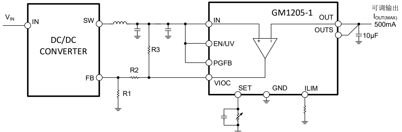
图 25. VIOC 典型应用
