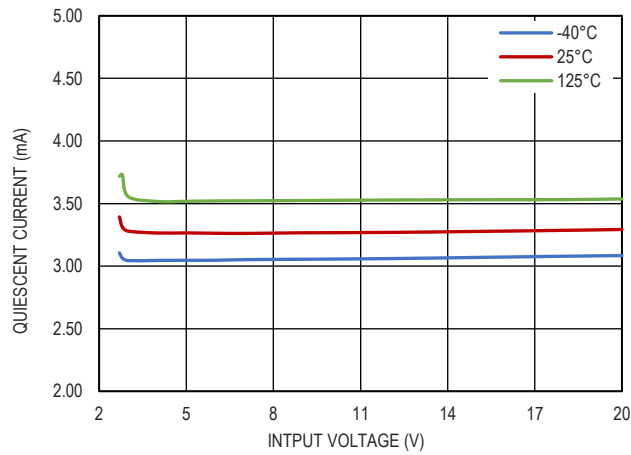
图 11. 静态电流和输入电压的关系, I_{OUT}=10\text{mA}
