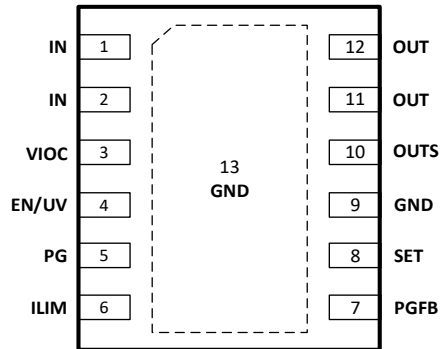
图 3. DFN12 (3mmx3mm GM1205ACPZ-2 和 4mmx4.9mm GM1205ACPZ-1 兼容 MSOP-12) 引脚配置(顶视图)
