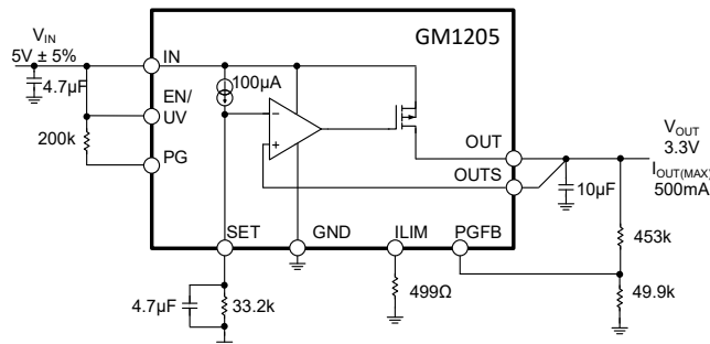
图 23 典型应用
