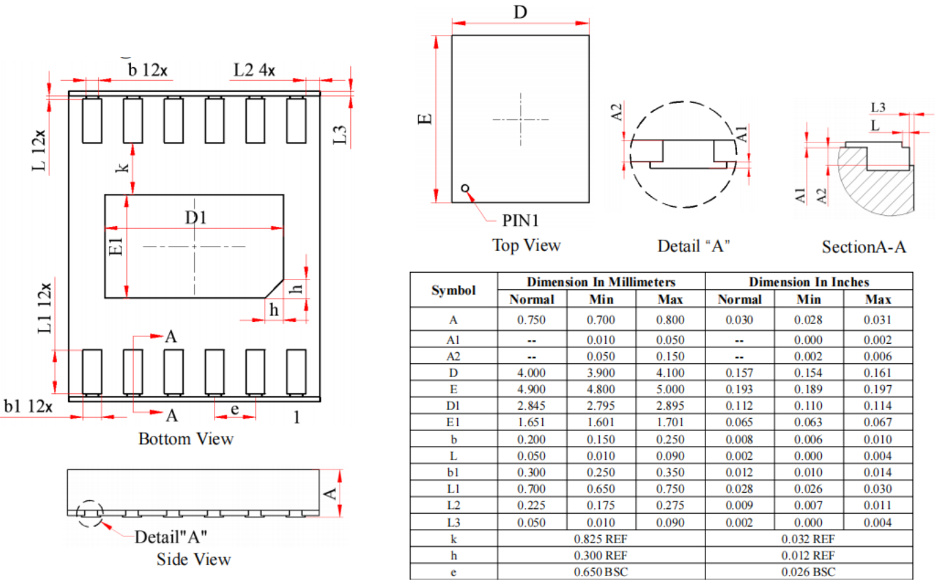
图 27. GM1205ACPZ-1-R7 和 GM1205ACPZ-3-R7 DFN12 封装 (4mmx4.9mm, CP-12-2) 和 MSOP-12 管脚兼容
