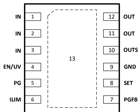
图 4. DFN12 (4mmx4.9mm GM1205ACPZ-3 兼容 MSOP-12) 引脚配置(顶视图)
