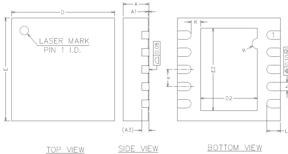
图 26. DFN10 封装 (3mmx3mm)
