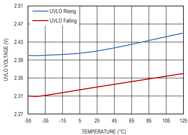
图 17. UVLO 阈值
