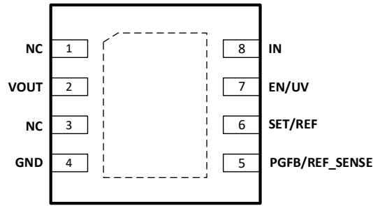
图 7. DFN8 (GM12051ACPZ-2)引脚配置(顶视图)
