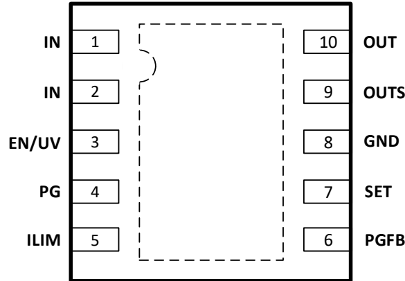
图 5. DFN10(GM12051ACPZ)引脚配置(顶视图)
