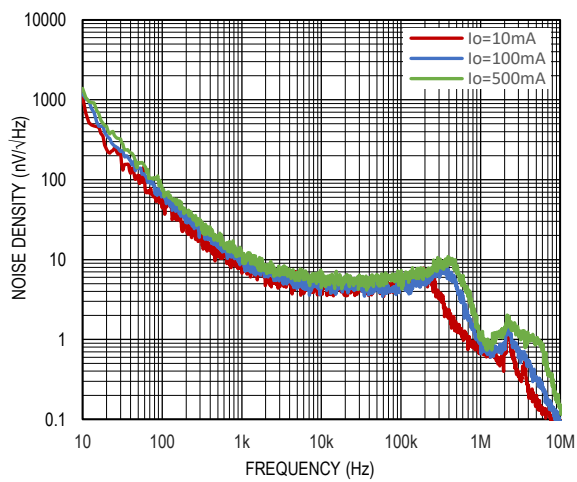
图 15. 输出噪声谱密度, V_{IN}=-4.3V , V_{OUT}=-3.3V
