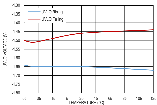
图 12. UVLO 阈值
