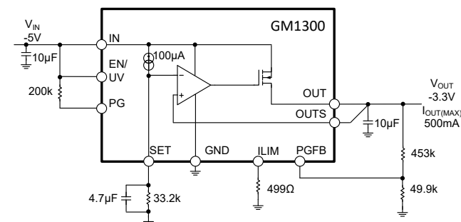
图 19. 输出电压稳压调节
