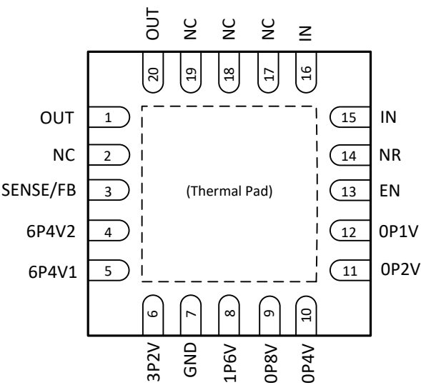
8 引脚 SOIC 图 2 引脚配置
