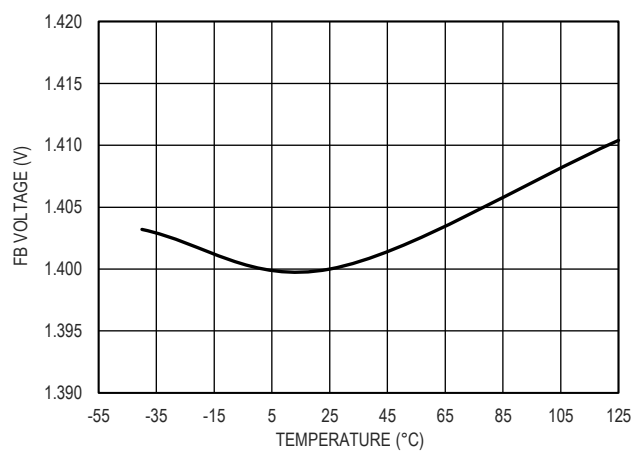
图 4. FB 引脚精度
