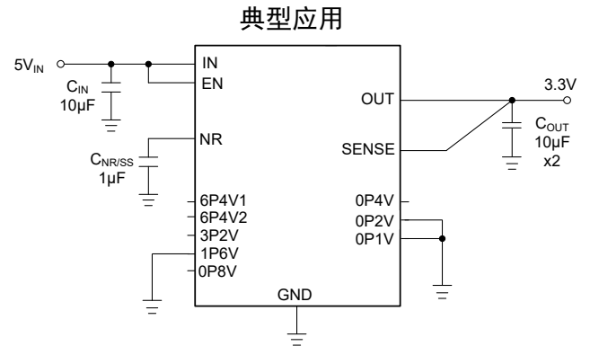
图 1 典型应用
