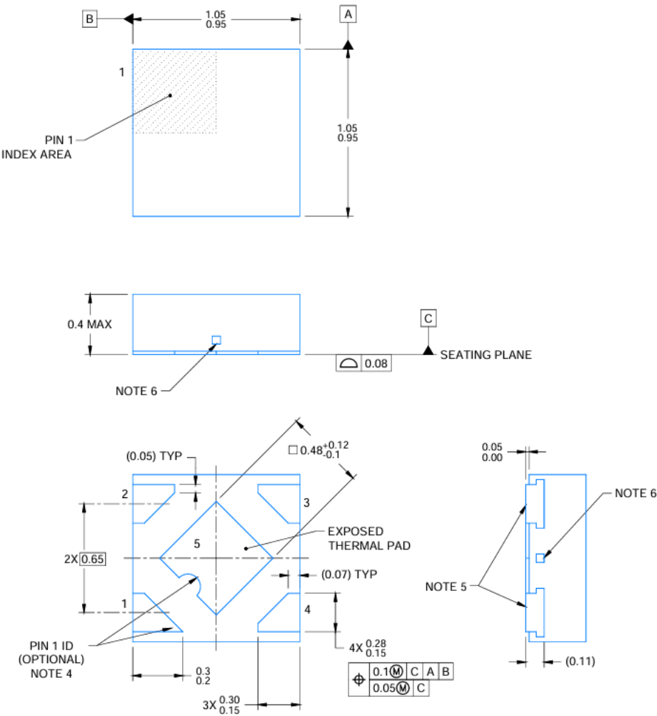
图 26.4 脚 DFN-4
