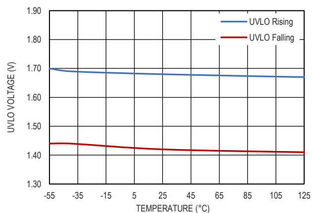
图 17. UVLO 阈值和温度的关系
