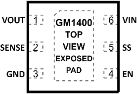
图 3.5 引脚 DFN-6 的引脚配置
