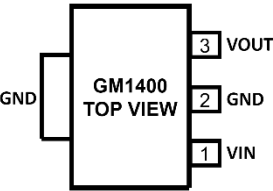
图 4.3 引脚 SOT-223 引脚配置
