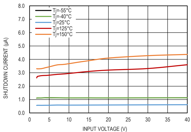
图 11. 关机电流和输入电压的关系
