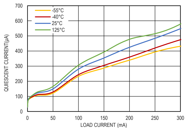
图 10. 静态电流和负载电流的关系, V_{IN}=4.3V
