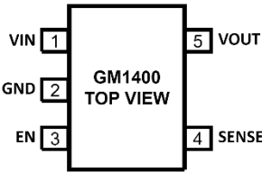
图 7.3 引脚 SOT-23 引脚配置
