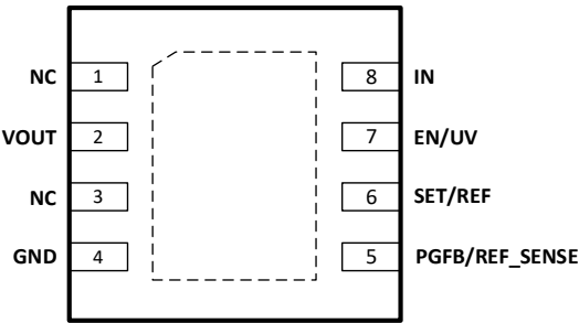
图 7. DFN8 (GM12051ACPZ-2)引脚配置(顶视图)
