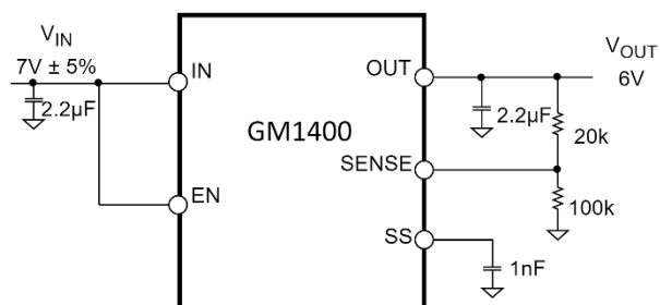
图 27. 典型可调输出电压应用原理图
