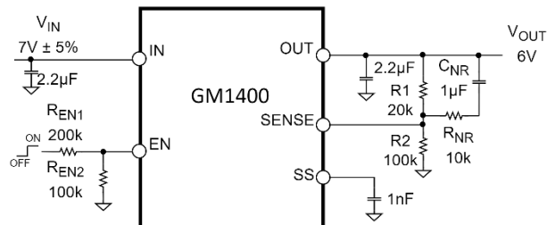
图 31. 噪声优化
