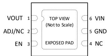
图 3. DFN6 引脚配置(顶视图)
