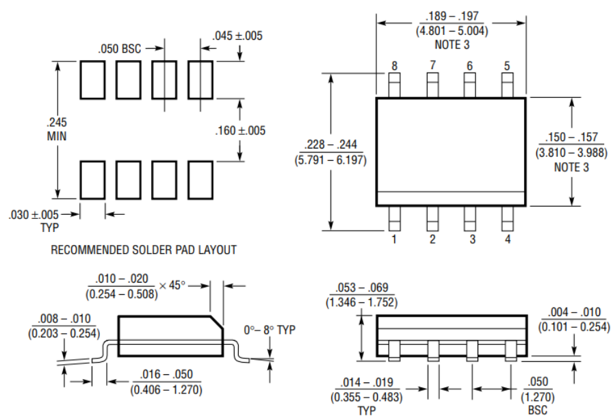
图 21. 8 引脚 SOIC-8
