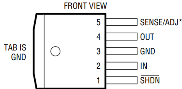
图 2 引脚配置
