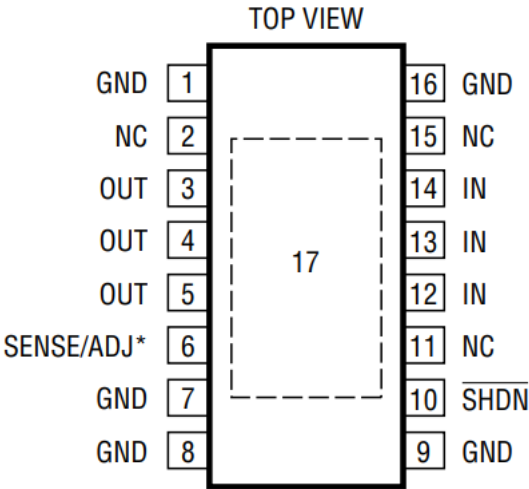
图 3 引脚配置
