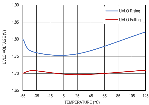
图 14. UVLO 阈值
