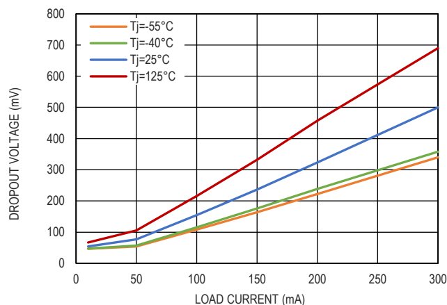
图 7. 3.0V 压差电压和负载电流的关系
