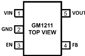
图 6.5 引脚 SOT-23 引脚配置（可调输出）
