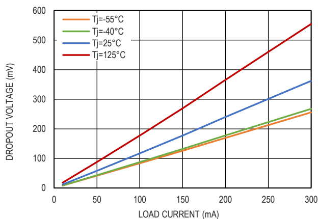
图 8. 7.0V 压差电压和负载电流的关系
