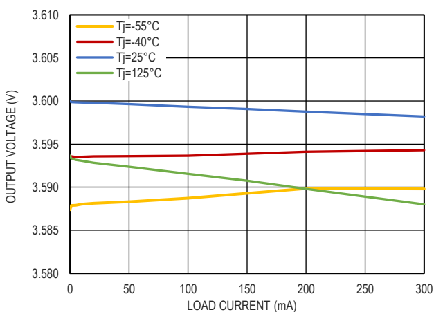
图 12. 3.6V 输出电压和负载电流的关系
