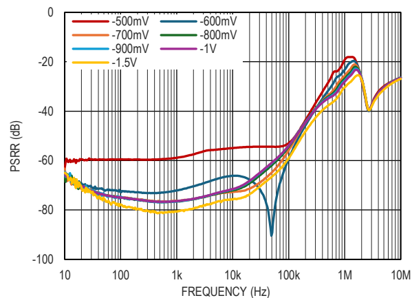
图 11. PSRR 和压差的关系, I_O = 500\text{mA}
