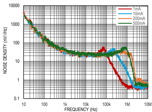
图 10. 噪声谱密度
