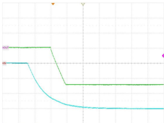
图 16. 软启动, V_{IN} = -6V , V_{OUT} = -5V , I_O = -500mA
