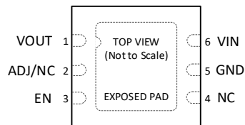
图 3. DFN6 引脚配置(顶视图)
