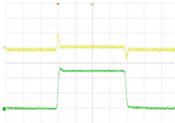
图 17. 负载瞬态响应, V_{IN} = -6V , V_{OUT} = -5V , I_O = -10 至 -500mA
