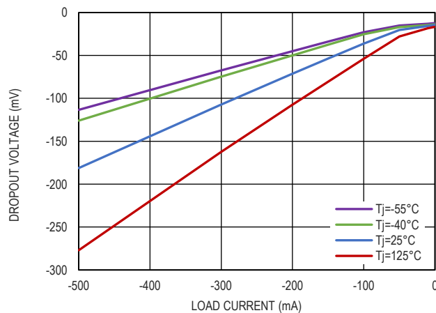
图 9. 压差电压和负载电流的关系
