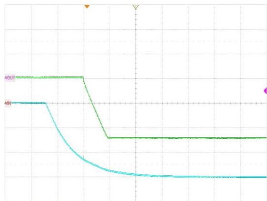
图 17. 软启动, V_{IN} = -6V , V_{OUT} = -5V , I_O = -500mA
