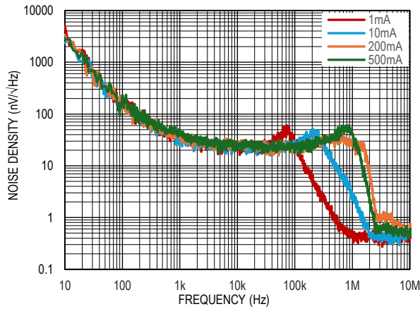
图 11. 噪声谱密度
