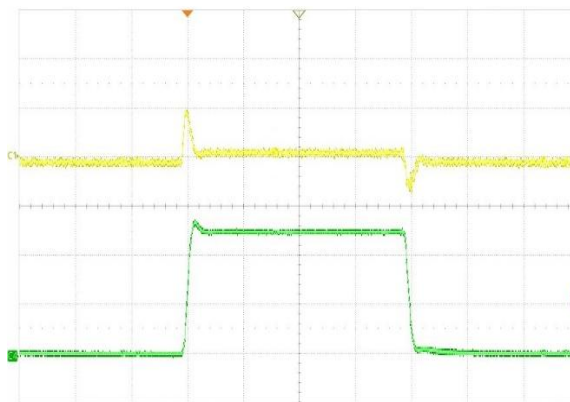
图 18. 负载瞬态响应, V_{IN} = -6V , V_{OUT} = -5V , I_O = -10 至 -500mA
