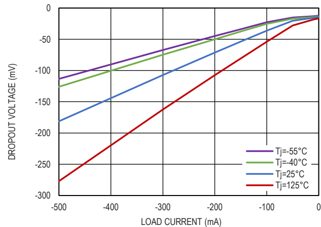
图 10. 压差电压和负载电流的关系
