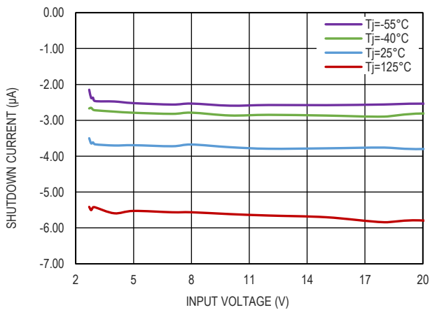
图 9. 静态电流与输入电压的关系
