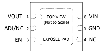
图 4. 2mm x 2mm DFN6 引脚配置(顶视图)
