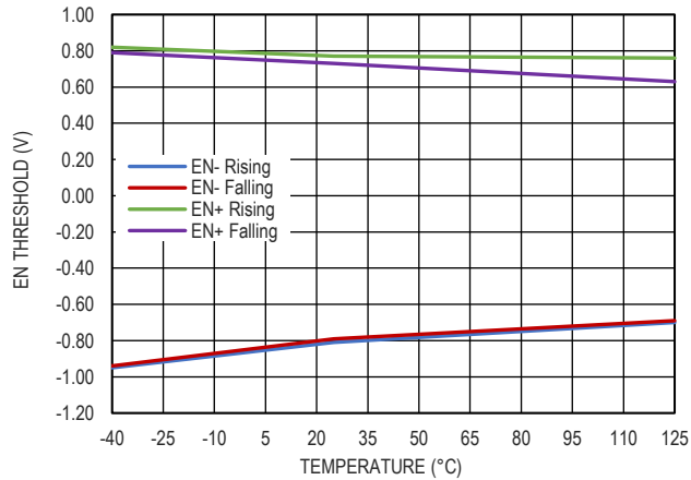
图 15. EN 阈值和结温的关系
