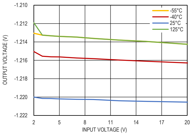
图 7. ADJ 引脚电压与 vs. 输入电压的关系
