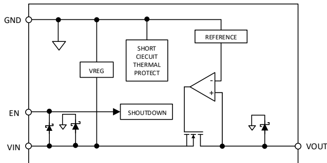
图 19. 固定输出电压内部框图
