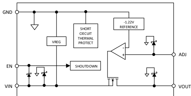
图 20. 可选输出电压型号内部框图
