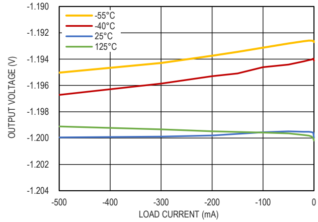
图 6. ADJ 引脚电压与 vs. 负载电流的关系
