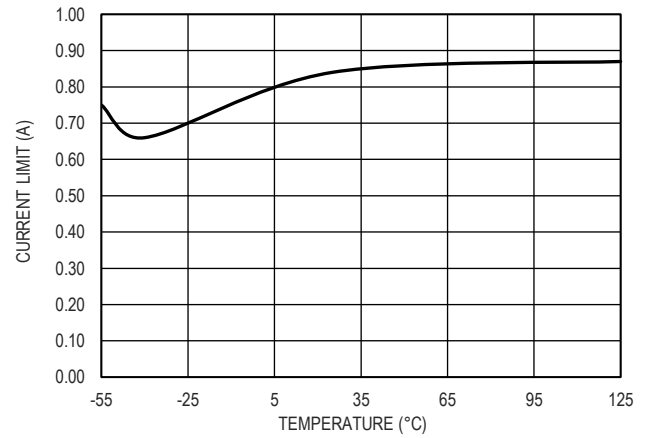
图 16. 限流值和结温的关系
