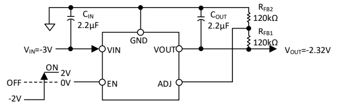
图 1 典型应用
