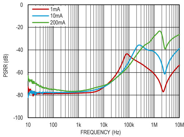
图 13. PSRR 和负载电流的关系
