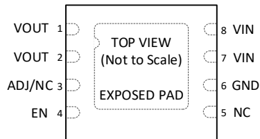
图 3. 3mm x 3mm DFN8 引脚配置(顶视图)
