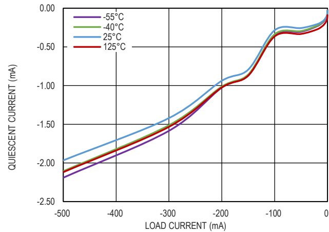
图 8. 静态电流与负载电流的关系
