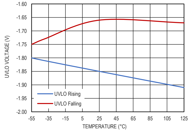
图 14. UVLO 阈值和结温的关系
