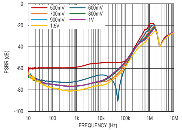
图 12. PSRR 和压差的关系, I_o = 500mA
