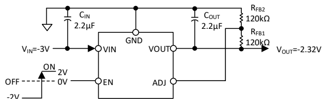
图 21. 设置可调输出电压
