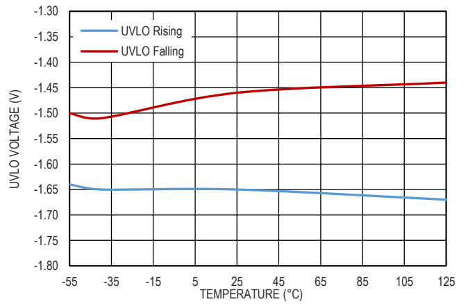
图 12. UVLO 阈值
