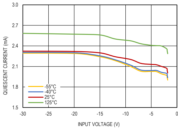
图 9. 静态电流和输入电压的关系, I_{OUT}=10mA
