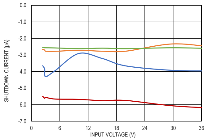
图 10. 停机静态电流和输入电压的关系
