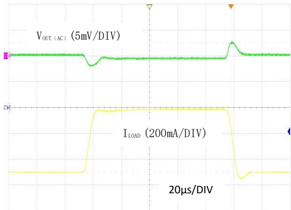
图 18. 负载瞬态响应, V_{IN}=-4.3V , V_{OUT}=-3.3V , I_{OUT}=10mA to 500mA
