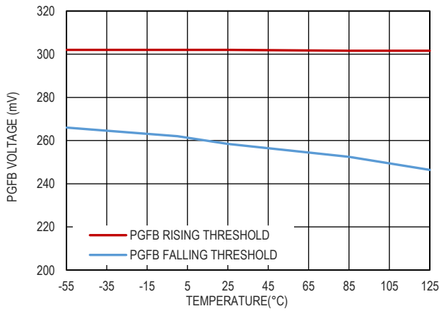
图 15. PGFB pin 阈值
