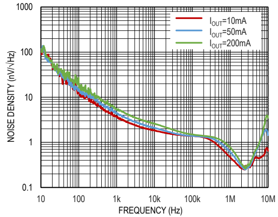
图 16. 输出噪声谱密度, V_{IN}=5V , V_{OUT}=3.3V
