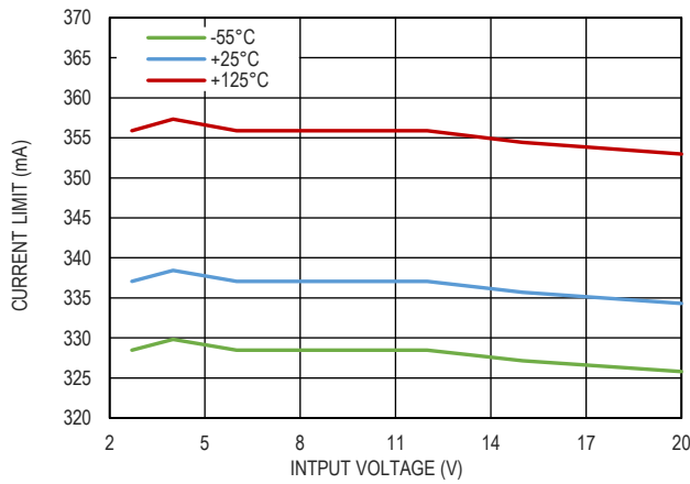
图 13. 输出限流值和输入电压的关系
