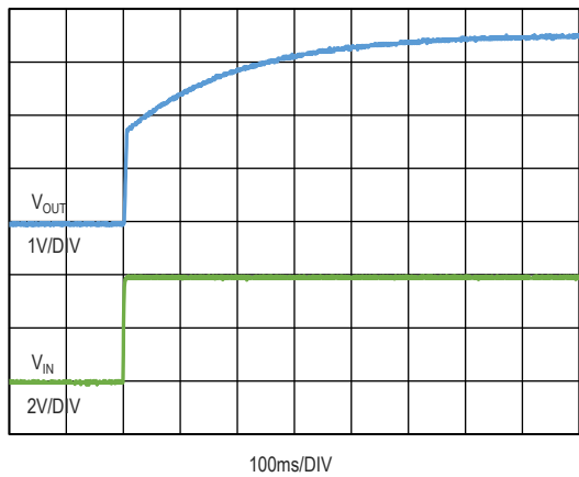
图 19. 软启动, V_{IN}=4V , V_{OUT}=3.3V , I_{OUT}=200mA
