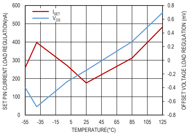
图 7. SET pin 电流、|V OUT -V SET |和温度的关系
