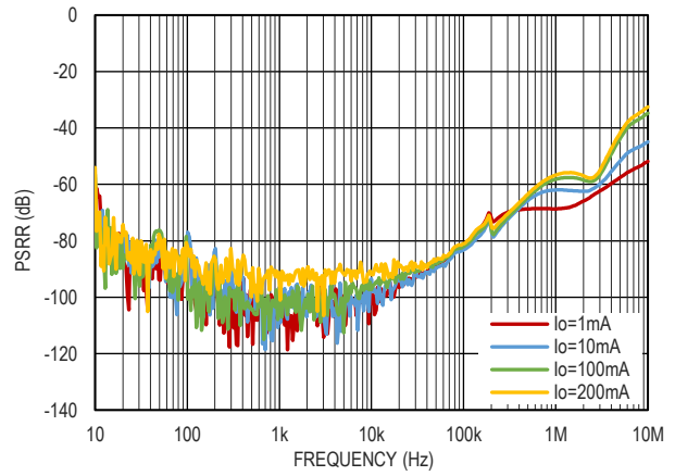
图 18. 电源电压纹波抑制比, V_{IN}=4.3V , V_{OUT}=3.3V
