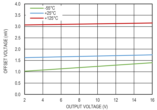
图 6. |V OUT -V SET |和输出电压的关系
