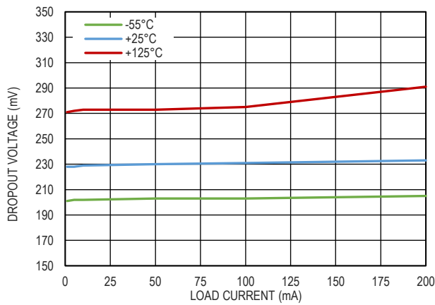
图 11. 压差电压和负载电流的关系, V_{OUT}=5.0V
