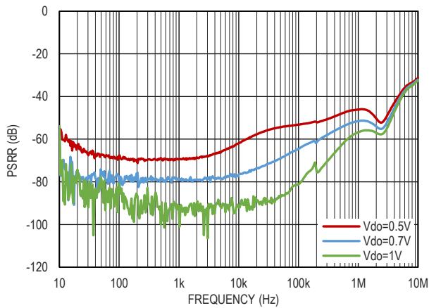
图 17. 电源电压纹波抑制比和压差的关系, I_{OUT}=200mA
